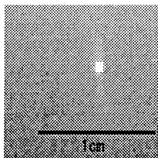
図 2: 小さいペンタノールの液滴を作ったとき。ほとんど変形していない。
