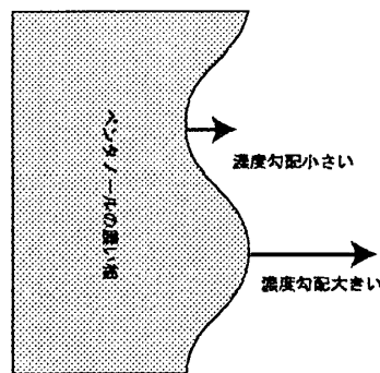
図 4: 矢印が界面張力の大きさを表す。矢印の大きさの差が \gamma_2
