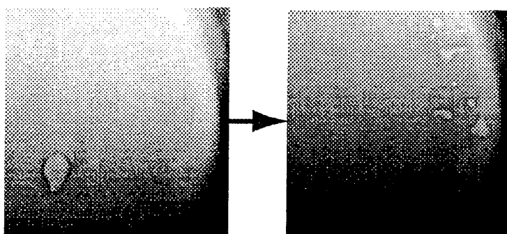
図 1: 大きいペンタノールの液滴を作ったとき。自発的に分裂していく。
