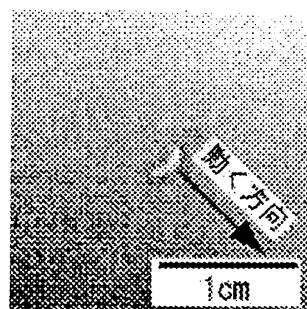
図 3: 中間の大きさの時。くの字になって動く。
