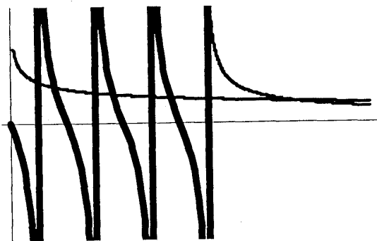
図 4. 振動準位の非線形性によるシフト
