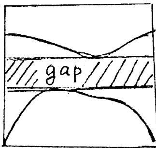
図 15. optical lattice のバンド構造
