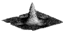
図 17. optical lattice における ILM の計算結果
