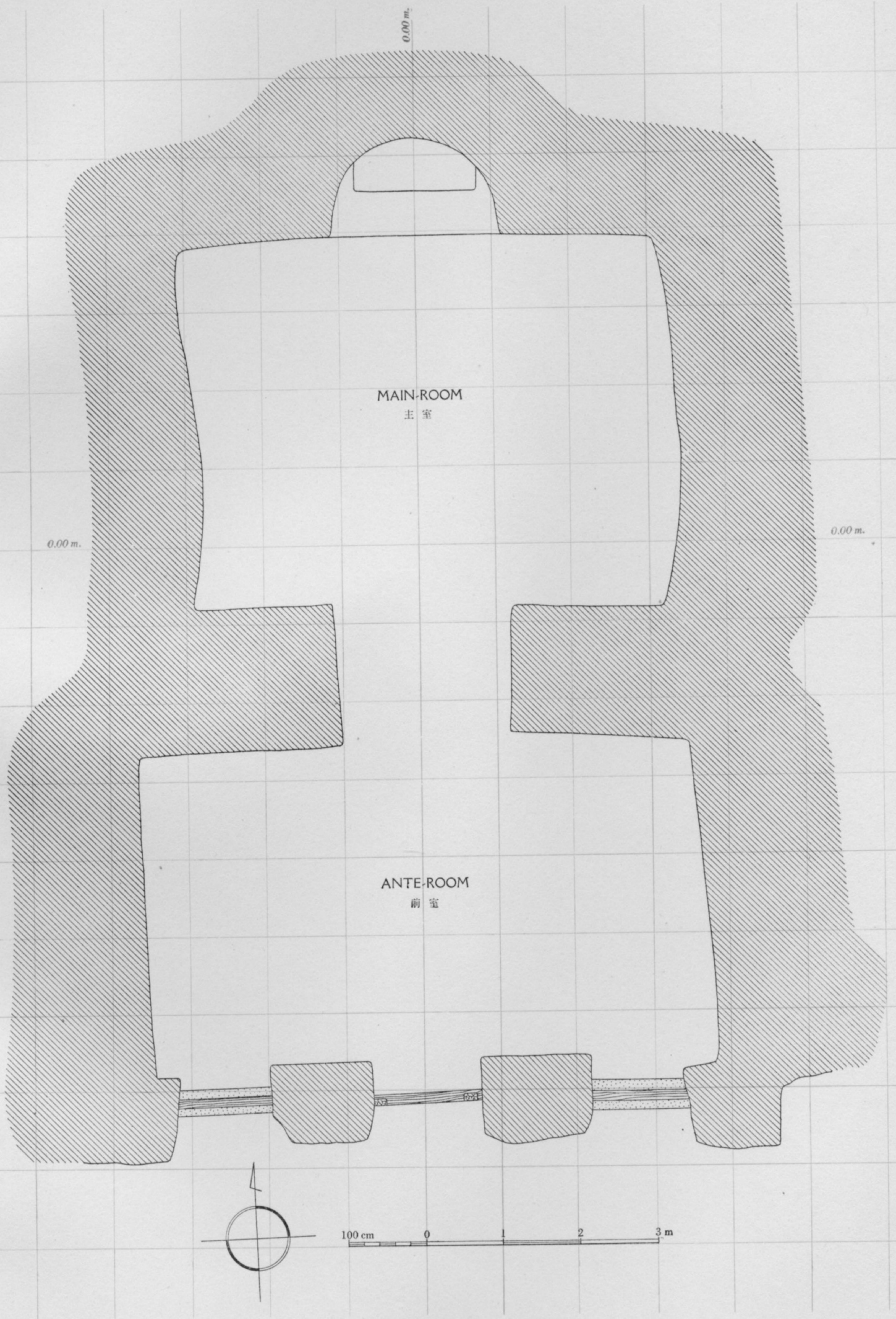
HORIZONTAL SECTION OF CAVE XII. 1:60 第十二洞 横断面图
