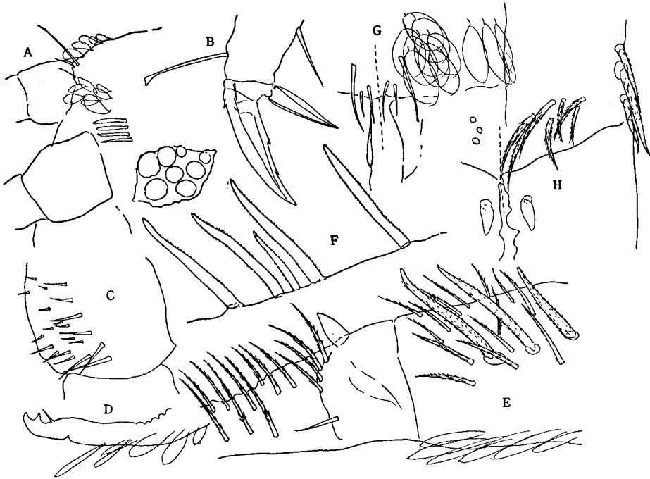
Fig. 18 Lepidocyrtus (Acrocyrtus) heterolepis sp. n.
