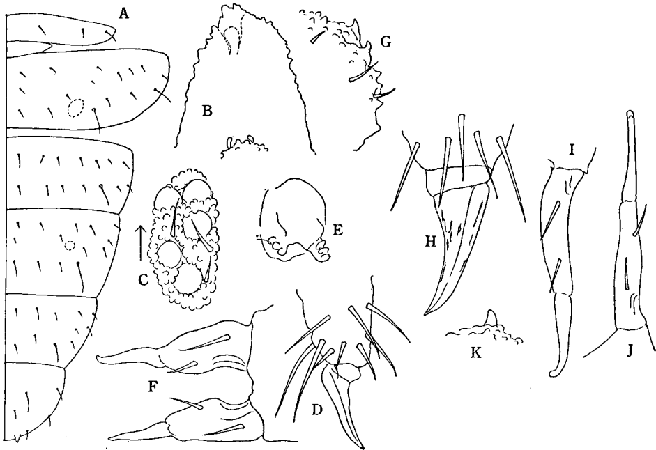
Fig. 2. Xenylla pseudobrevicaudata RITTER
