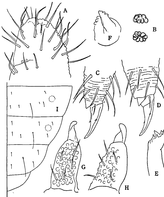
Fig. 3 Brachystomella contorta DENIS
