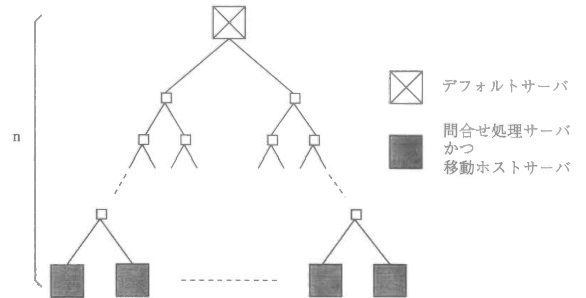
図2.6: 2分木トポロジ
