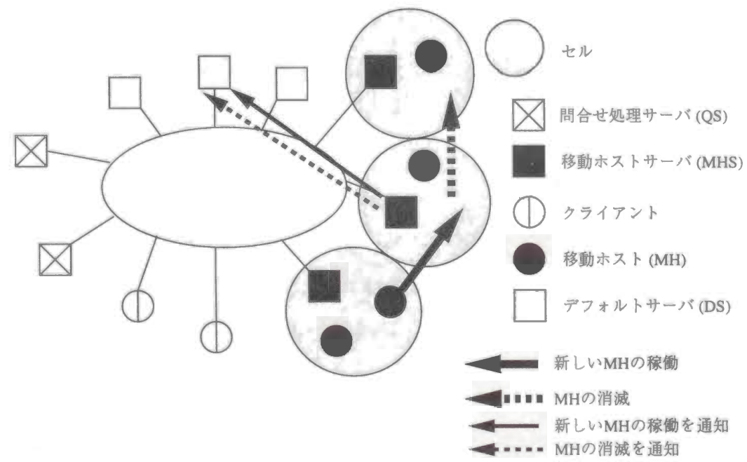
図 1.6: WDN の例
