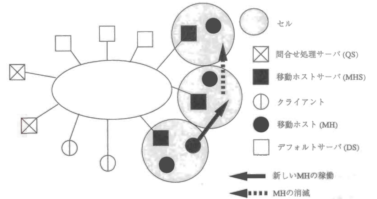
図 1.7: NN の例
