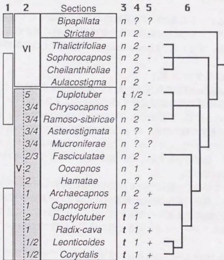
図V-5. Corydalis (キケマン属)の各sectionにおける種皮(表II-2)と果実(表III-3)の変異と、塊茎の有無・子葉の数・倍数化の有無。さらにrDNAのITS領域の塩基配列から推定した系統樹(Lidén & al. 1995, 図V-2)を重ね合わせた。
