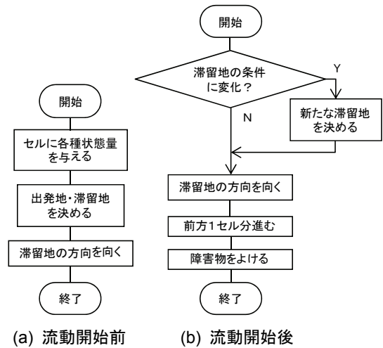
fig.6-16 エージェントのルールのフロー
