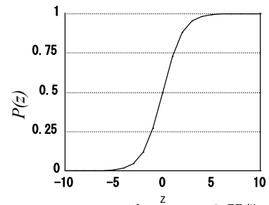
fig.8-9 ロジスティック関数
