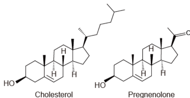
図 A Cholesterol(左)、Pregnenolone(右)の化学構造式
