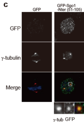
図22 P5はSgo1のN末端のコイルドコイル領域に直接結合する (A) MBP-Sgo1-Nter、Sgo1-Nter変異体の略図。 (B) MBPプルダウンアッセイ。精製タンパク質 (1 \mu g) とFITC-P5またはFITC-chol(100 \mu M)を18時間インキュベーションしamirose resin beadsで3時間プルダウンする。Beadsを洗浄後、535nmで蛍光強度を測定した。(mean \pm s.e.m. 3回のデータを用いてダネットの多重比較を行った (** p < 0.01 **** p < 0.0001) 担当；東浦、小田、松村 CBB染色はBeadsに結合しているタンパク量を示す。 (C) GFP-Sgo1-Nter (51-105) の細胞内局在 担当；松村
