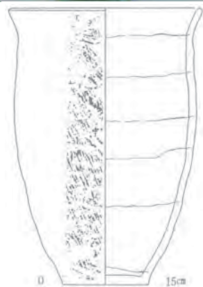
(土器実測図 : S=1/6)
