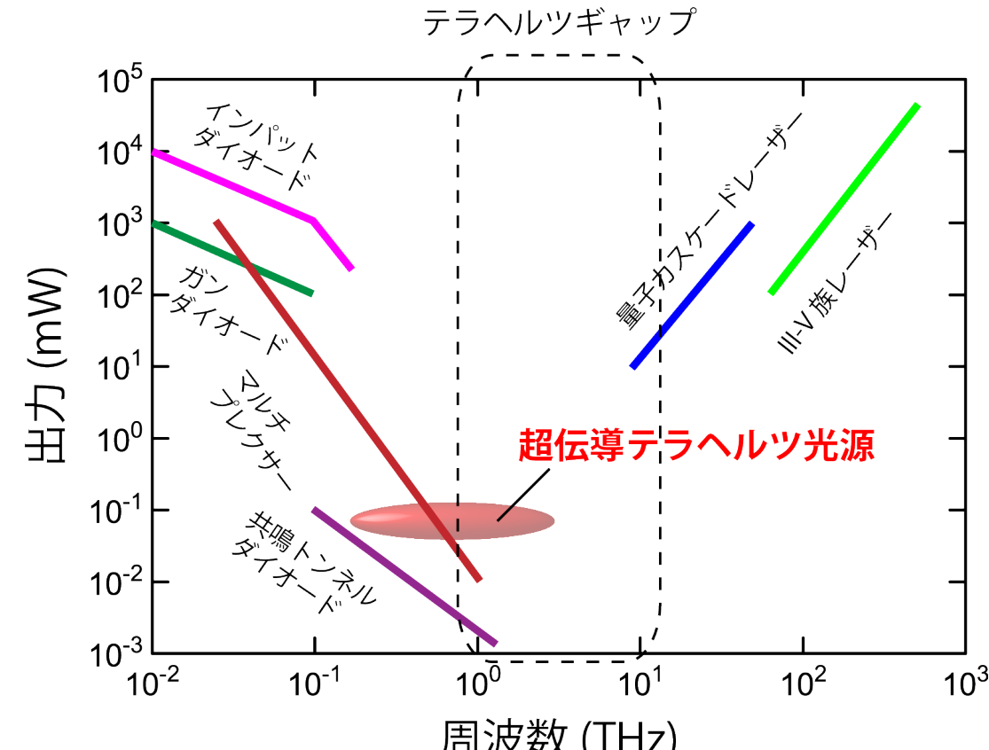
さまざまな連続テラヘルツ光源の周波数 vs. 出力プロット [2]
