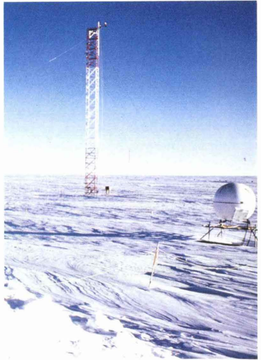
写真1 南極昭和基地の南約300km、標高2,230mのみずほ基地に建てられた30mの気象境界層観測用鉄塔
