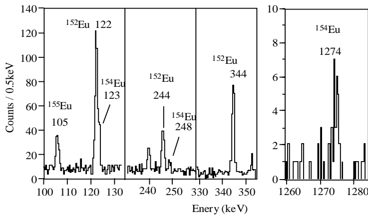
Fig. 5 10gの酸化ユウロピウム試薬中の ^{152}\text{Eu} ^{154}\text{Eu} ^{155}\text{Eu} の検出
