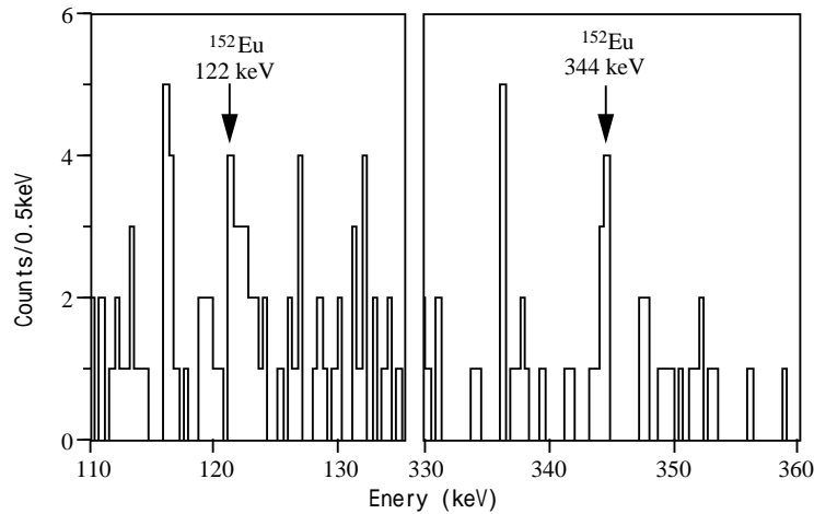
Fig. 4 1gの酸化ユウロピウム試薬の測定による ^{152}\text{Eu} の発見
