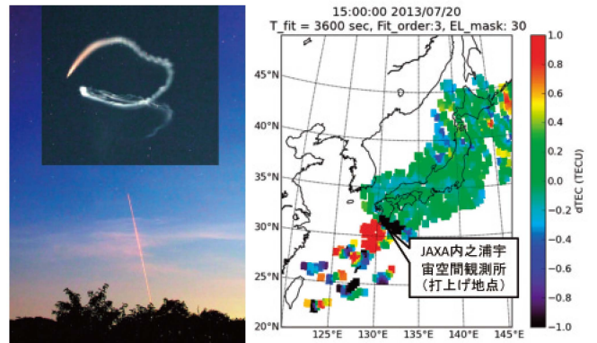
[左] 観測ロケット上昇とTMA発光雲（せんだい宇宙館・早水氏および安藤氏提供） [右] GPS網によるロケット実験時の電離圏電子密度の水平分布（電子航法研・斉藤氏提供）
