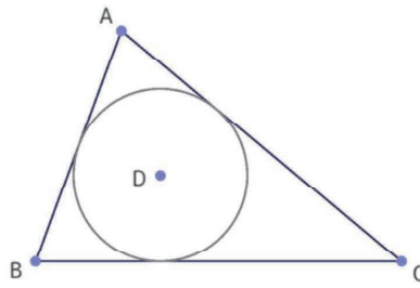
図3：三角形ABCとその内接円
