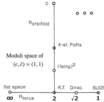
図 1: (1, 1) モジュライ空間
