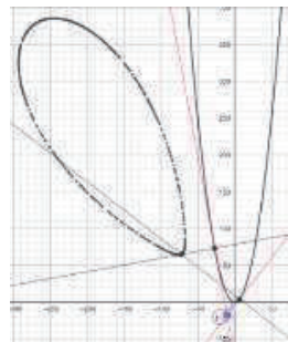
図8. 放物線 y=x^2/10
