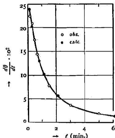
Fig. 7.—Expt. 6.
