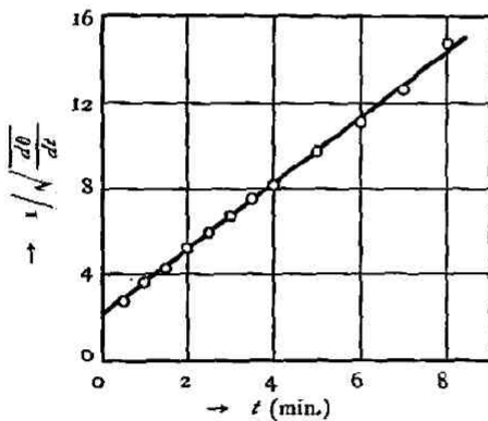
Fig. 3.—Expt. 4.
