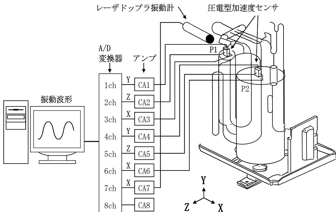
図5.6 振動測定装置
