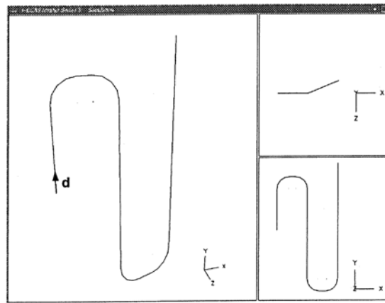
図4.33 配管3次元形状モデル(部品②)
