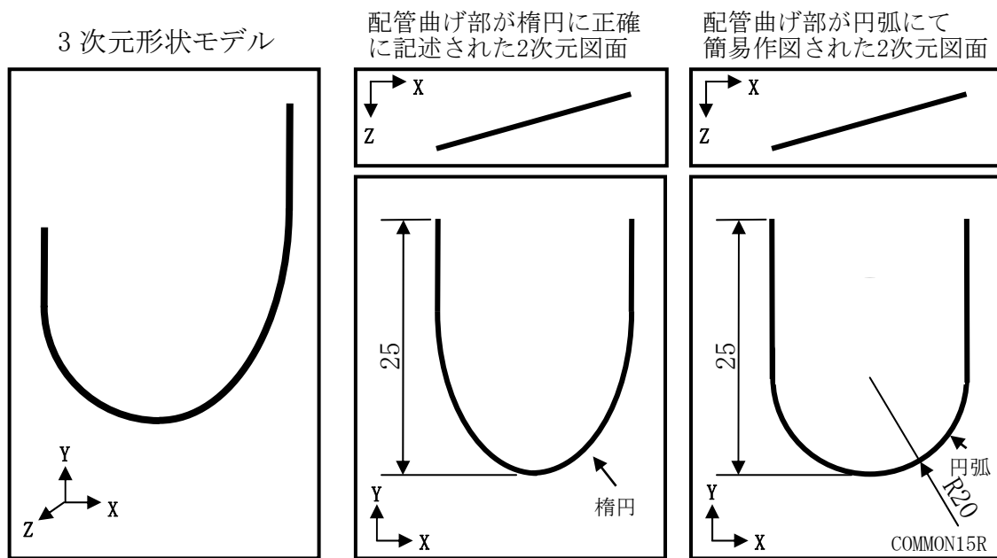
図4.16 配管2次元図面の簡易作図
