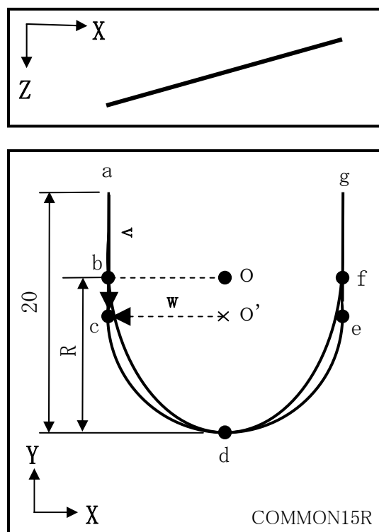
図4.19 配管2次元図面(2直線が平行の場合)
