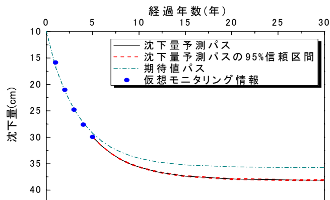
図-3.13 5年度における沈下量予測結果
