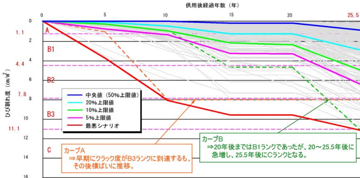
図-2.20 設計パフォーマンスカーブ
