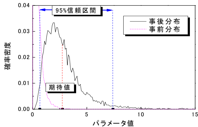
図-3.12 パラメータ \phi_{73} の事後分布
