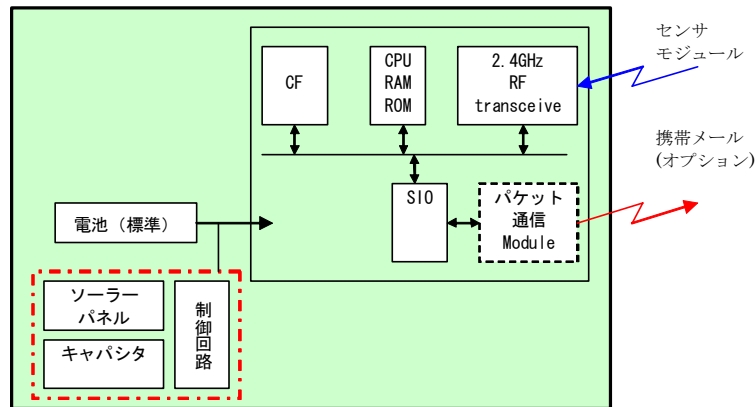
図 3.12 ゲートウェイユニットブロック図
