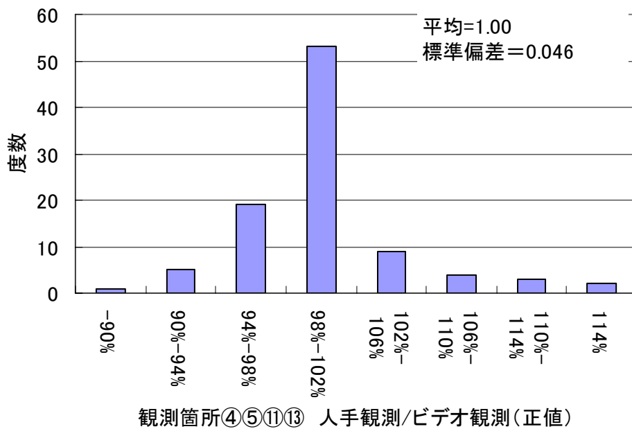
図 3.3 人手観測とビデオ観測（正值）との比の分布（観測箇所④、⑤、⑪、⑬）
