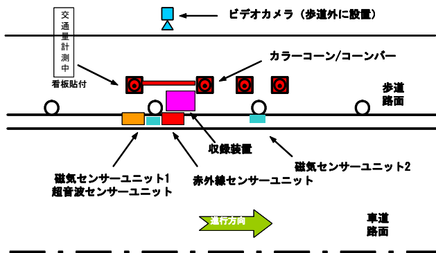
図 3.6 各センサの設置状況
