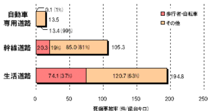
図 6.1 道路種類別の死傷事故率の比較（2004年） 4,3)
