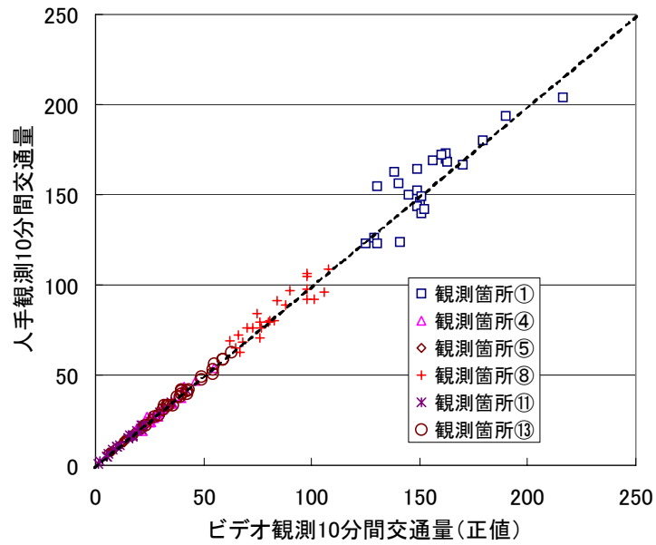
図 3.2 人手観測とビデオ観測（正值）との差
