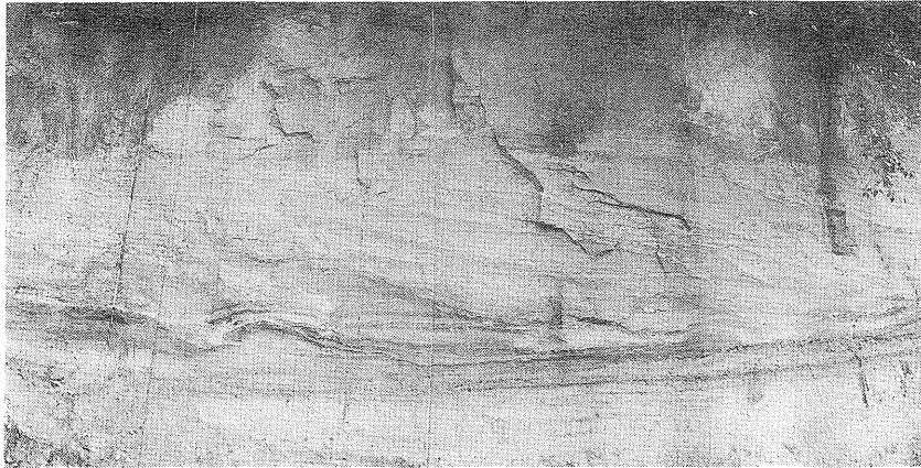
第6図 傾斜したユニットをなす逆級化層理. 地点2. スケールは5 m.
