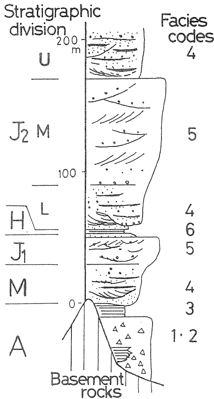
第3図 宇治丘陵の大阪層群模式層序と堆積相(堆積相区分は城陽礫層研究グループ, 1991). A: 青谷粘土・礫層, M: 明星ヶ原砂層, J 1 : 城陽礫層 I, H: 長谷粘土層, J 2 : 城陽礫層 II. 数字は堆積相区分.
