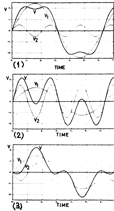
図5. 1:3同期による2重モード振動(5次特性)
