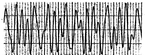
オ6図 四重モード振動波形の一例(アナログ計算機による) [10] [\delta=0, p_j=3.2]
