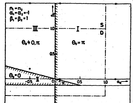
オ10図 発振器の結合系の同期領域 [12]
