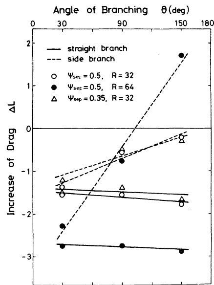
図9. 分岐による抵抗増加(モデル2)
