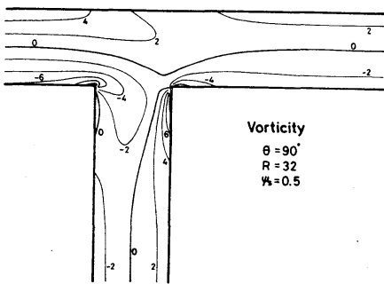
圖 4 等渦線 ( R=32, \psi_s=0.5 )
