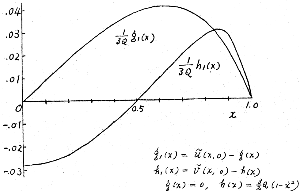
図 3. 出口においてはじめて設定したポアズイユの流速分布からのずれ。
