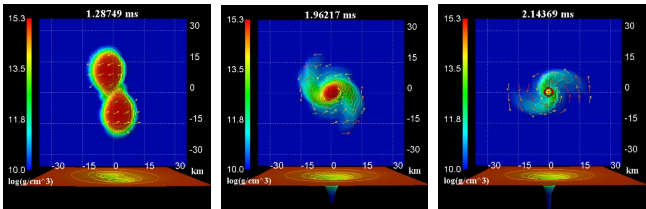
連星中性子星が合体し、最終的にブラックホールが生成される様子。最後の図の中心部分の赤い円は、そこにブラックホール地平面が形成されたことを表している。
