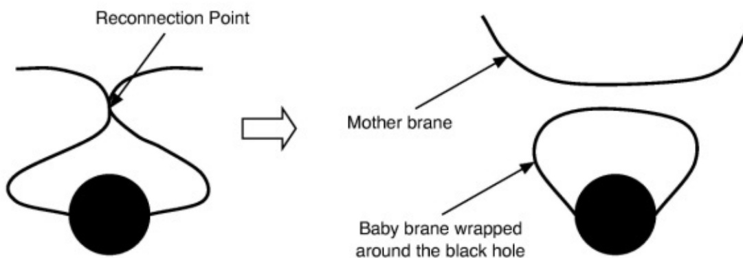
膜宇宙上に生成されたブラックホールが余剰次元方向へ落下する際に、ブラックホールがブレーンを引き折り新たに小さな膜宇宙が誕生する様子。
