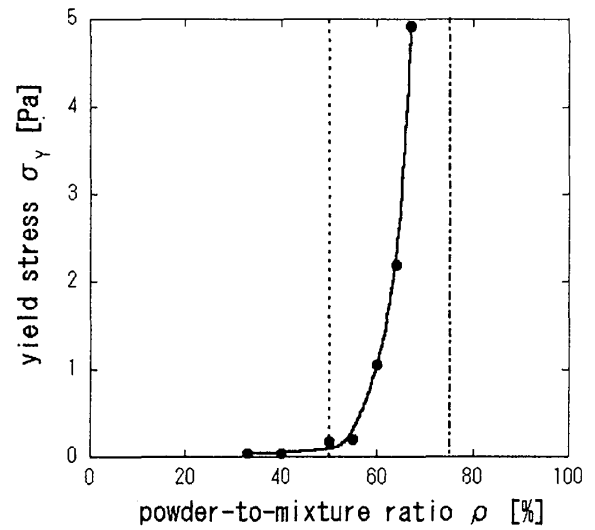
図4：降伏応力
