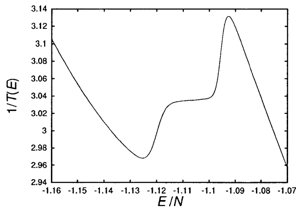
図 1: 単純立方格子 ( 20 \times 20 \times 20 , 周期的境界条件) 上のハイゼンベルク反強磁性模型についてのマイクロカノニカルな温度の計算結果。相互作用の大きさは最近接スピ間が J_1 = 1 、次近接スピ間が J_2 = 0.26J_1 で、いずれも反強磁性的とした。
