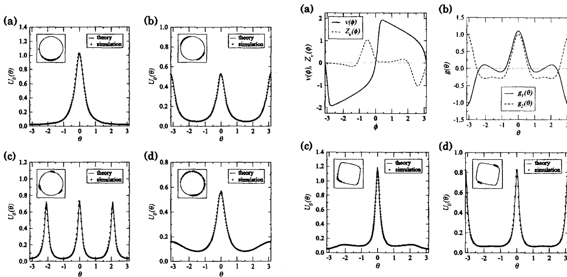
FitzHugh-南雲振動子の結果. (a) v(\phi) と Z_v(\phi) , (b) g_1(\theta) と g_2(\theta) , (c) 同期状態, (d) 2 クラスタ状態.
