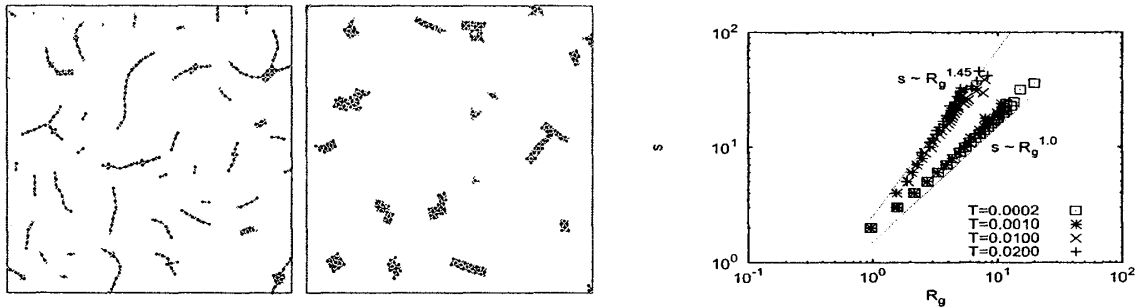
図 1: \phi = 0.04 における凝集過程のクラスター (系の一部を表示)。 T = 0.0010 (左) 及び T = 0.0200 (右)。 図 2: 回転半径 R_g のクラスターサイズ依存性。
