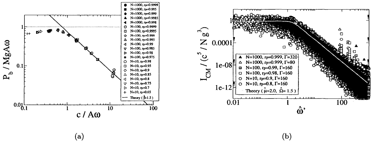
図1: (a) 異なる N , r_p , \Gamma ( \Gamma は 10~640 の範囲で変えた) について、無次元化されたエネルギー流入量 P_b を熱速度 c と最大振動板速度 A\omega の比の関数としてプロットしたもの。実線は \hat{\beta} = 1.5 としたときの理論の予測 ((5) 式の近似的等式)。 (b) 異なる N , r_p , \Gamma についての無次元化された重心高さのパワースペクトル。灰色の太線は \hat{\mu} = 2.0 , \hat{\Omega} = 1.5 としたときの理論曲線 ((6) 式第2項)。
