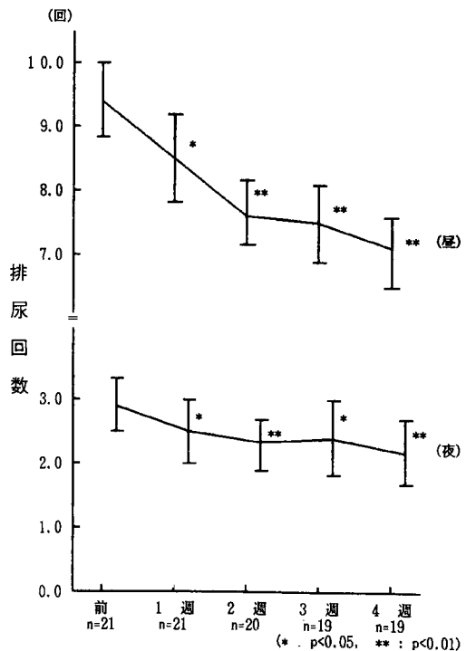
Fig. 2. 排尿回数の推移
