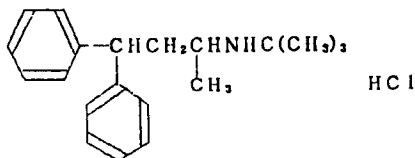
Fig. 1. 構造式
