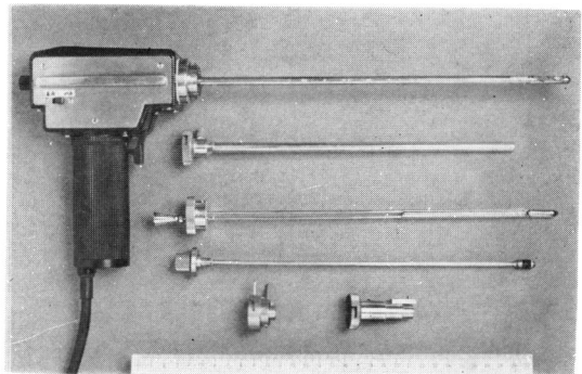
Fig. 1. 経尿道走査用スキャナー。その外套管、男性用および女性用オプチュレータ。手術用膀胱鏡外套管に接続するためのアダプター(二種)
