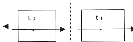
図 5 = 例(386) c.
