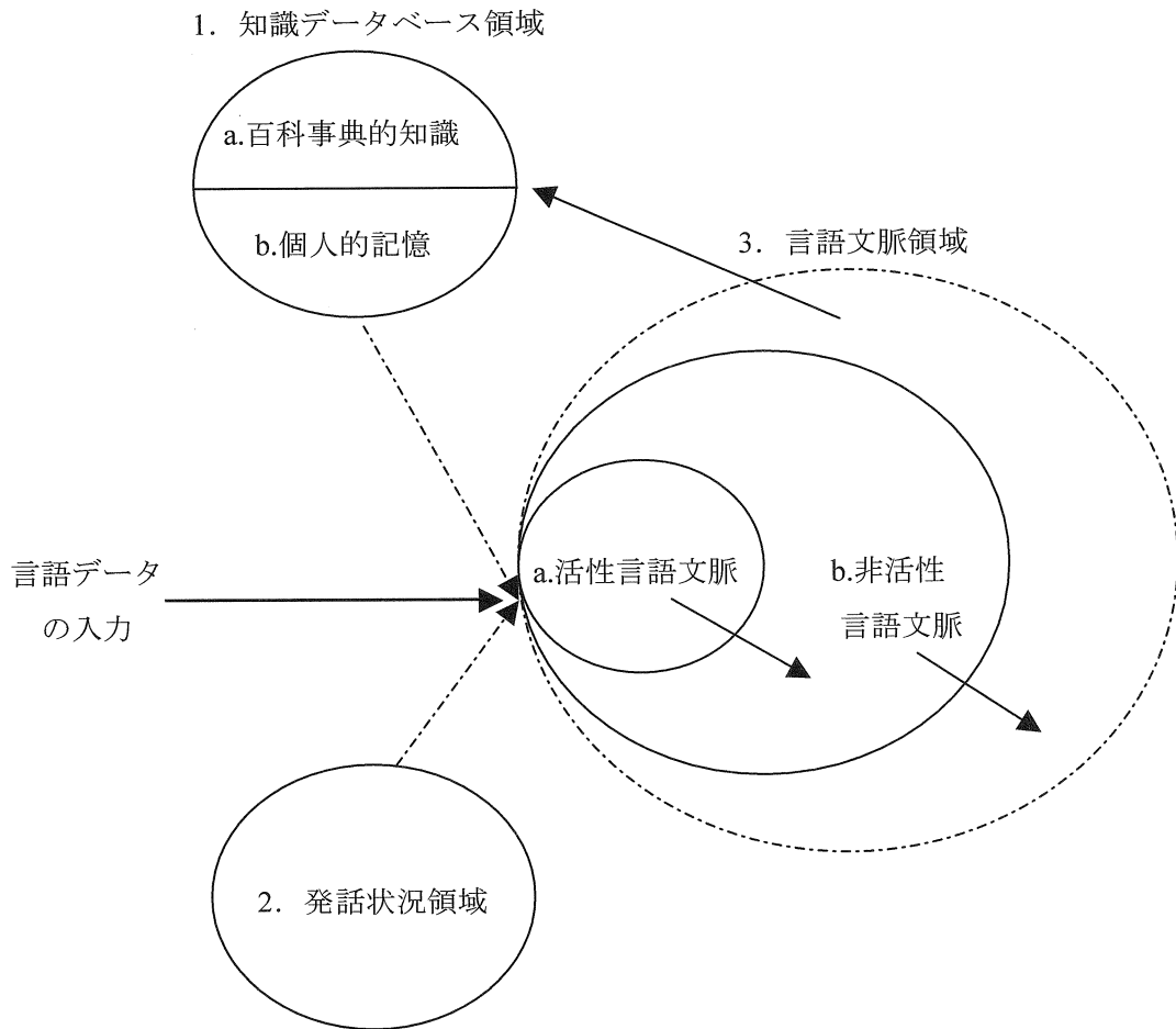
図3 談話モデル 61
