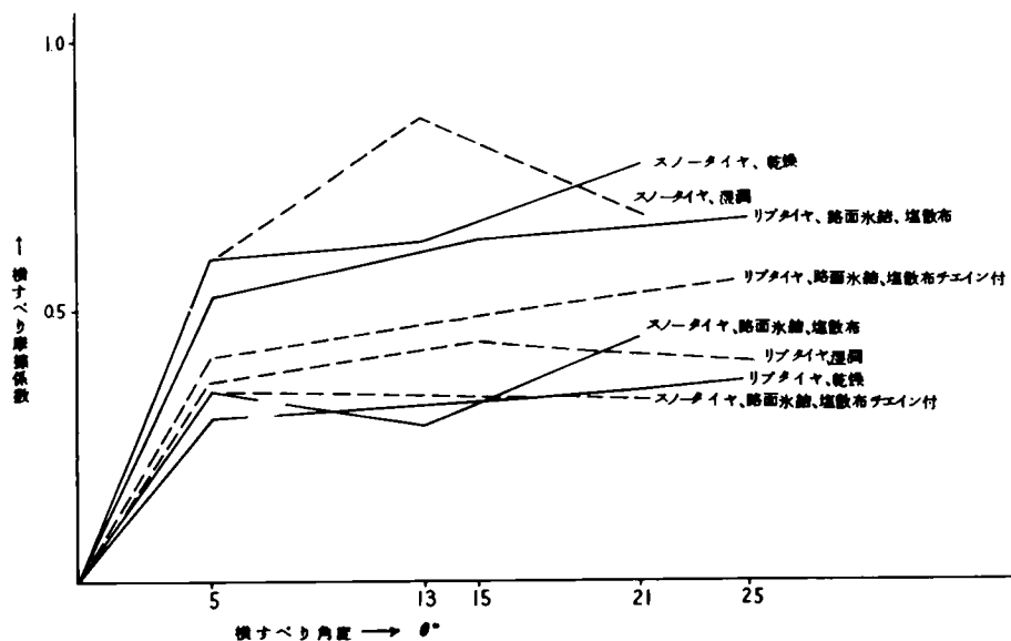
図 4-45 横すべり角と横すべり摩擦係数 (密粒アスコン、 20 \text{ kN/m}^2 )
