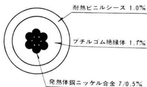
図7-16(a) ゴム被覆電熱線
