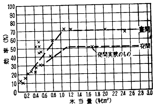
図7-19 1回降雪量と効率の関係
