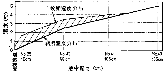
図 7-23 地中温度上昇図
