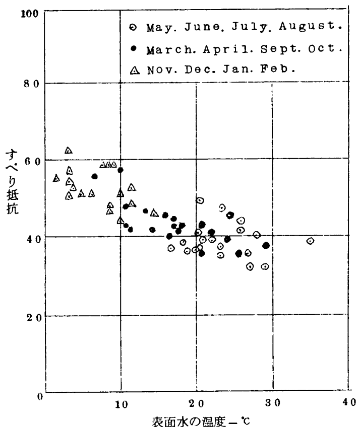
図4-22 温度および季節と摩擦係数
