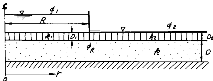
図-5.14 浸透条件 (c-i)
