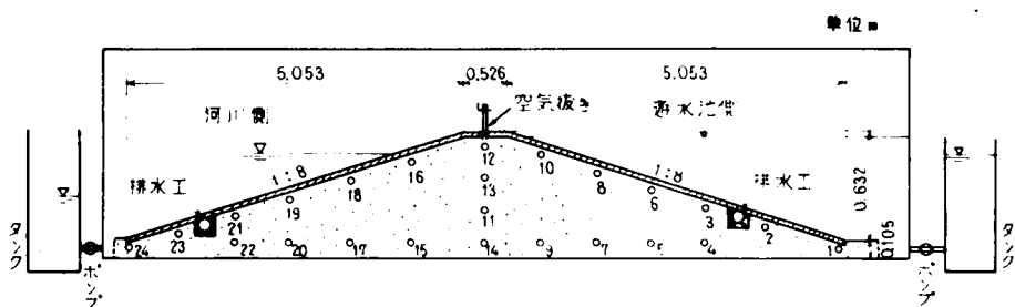
図-8.12 砂模型実験装置
