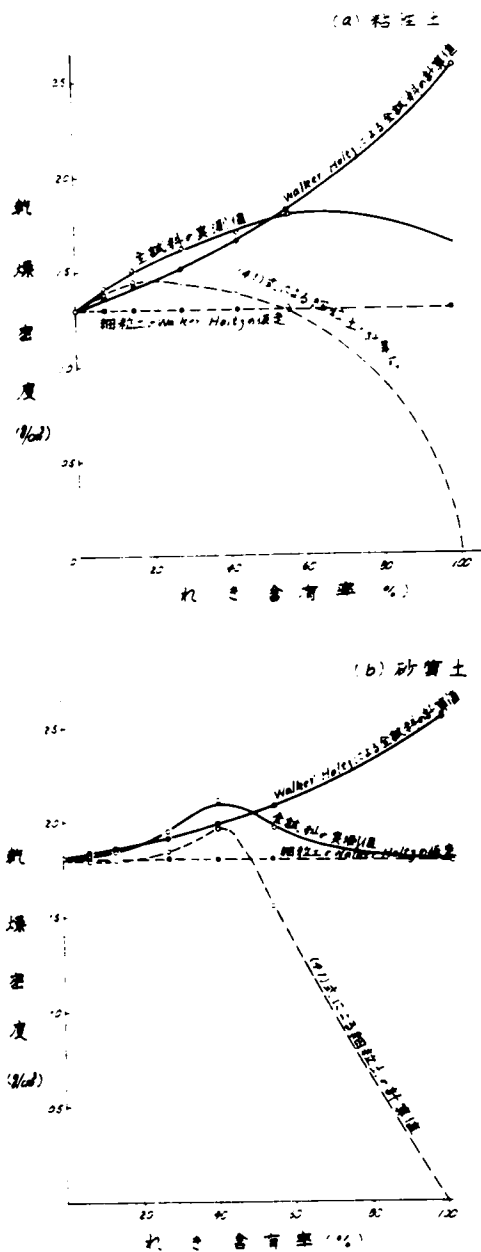
図-4.6 乾燥密度とれきの含有率(れきを粒径5mm以上とする)
