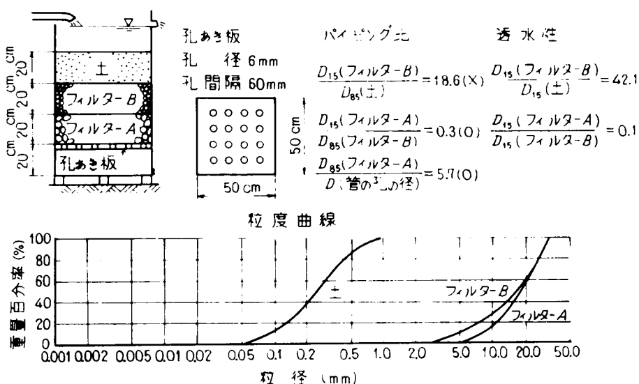
図- 8.2 3 孔あき板を用いたフィルターの実験の1例
