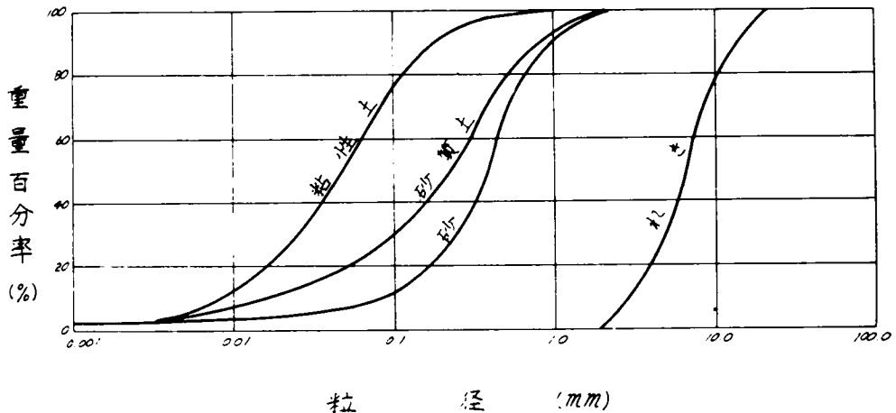
図-4.1 試料の粒度曲線
