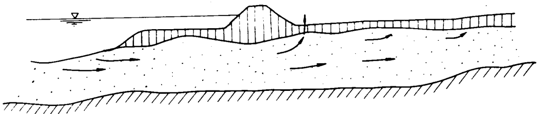
図-5.1 代表的な地盤漏水
