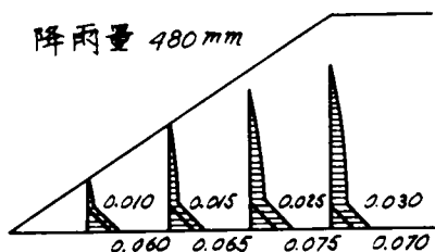
図-7.18 盛土内の間げき圧の分布
