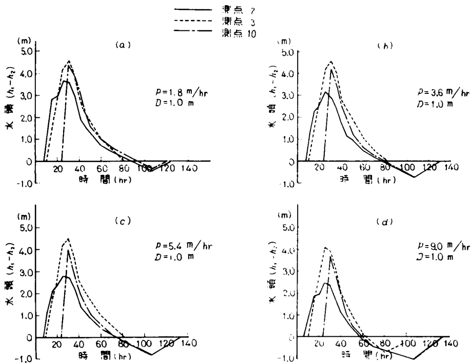
図-8.14 フェイシングに作用する水頭
