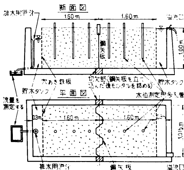
図-6.9 実験に用いた水槽
