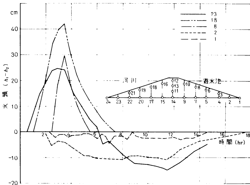
図-8.17 フェイシングに作用する水頭（砂模型の実験結果の1例）
