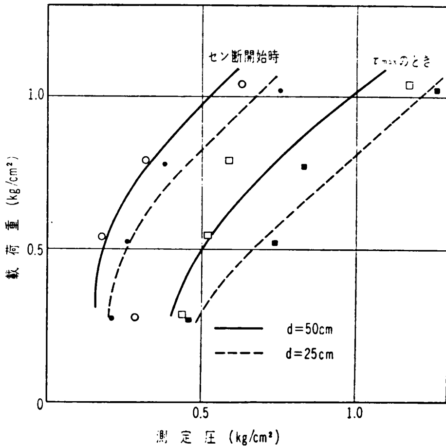
図-4.19 載重と測定圧の関係
