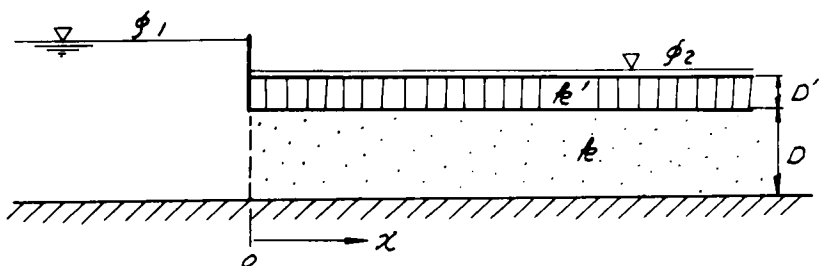
図-5.2 浸透条件 (a-i)
