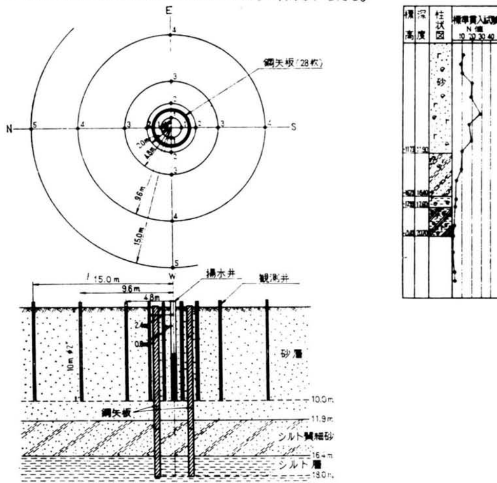
図 - 6.2.2 地盤の成層状態ならびに平面図
