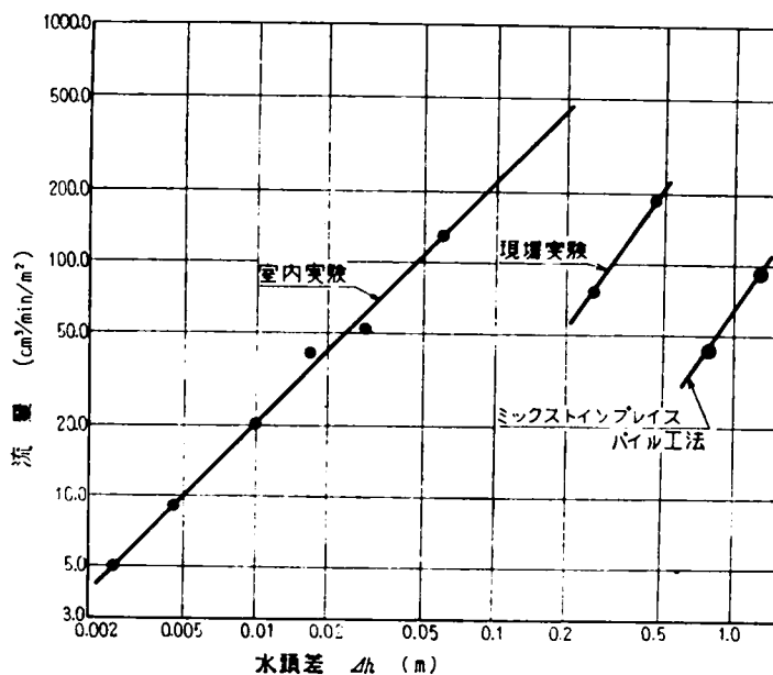
図一 6. 2 6 現場に施工した止水壁の効果と室内実験結果との比較
