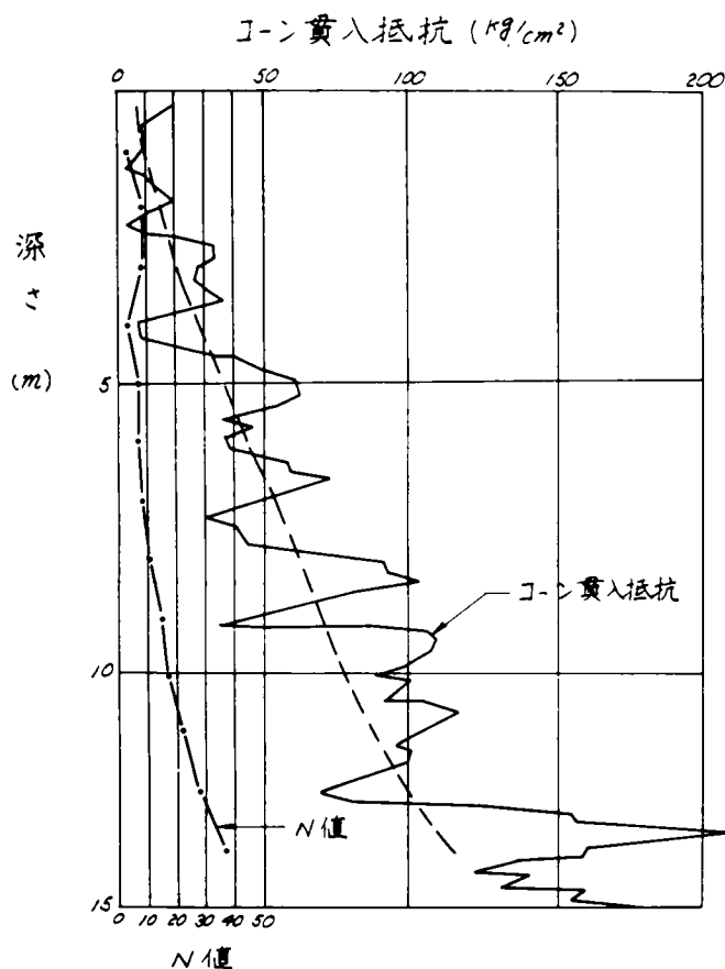
図-2.12 コーン貫入抵抗とN値の比較の1例
