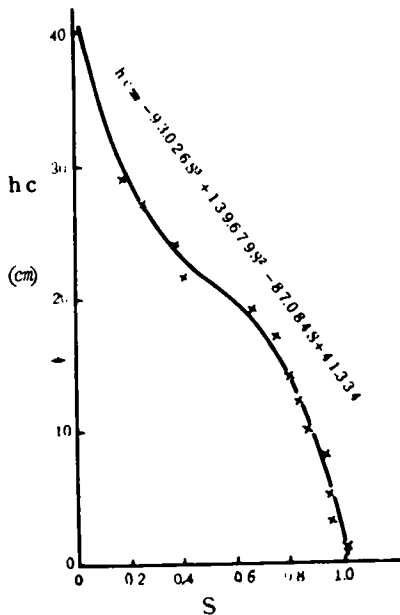
図-7.11 飽和度と毛管水頭の関係
