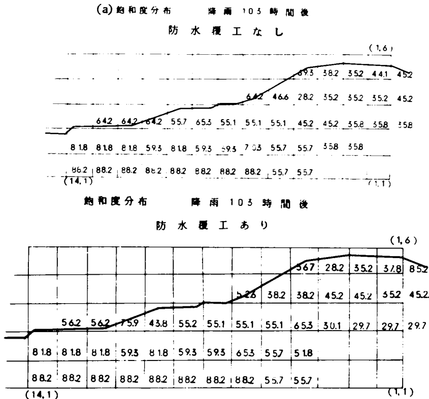
図-7.7 堤体内の飽和度分布の1例
