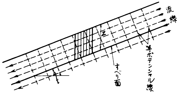
図-2.9 浸透流と地震が作用したときのり面
