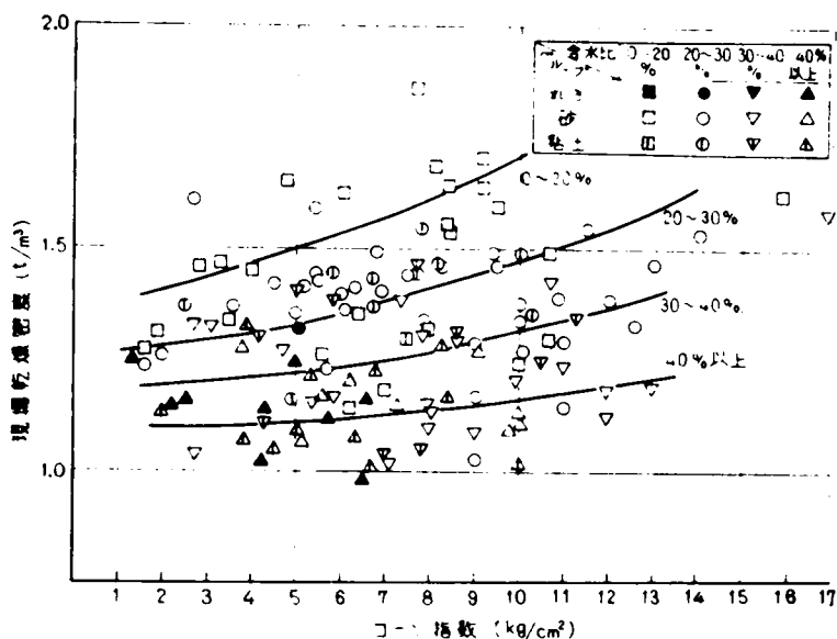
図-3.1.1 現場乾燥密度とコーン指数の関係
