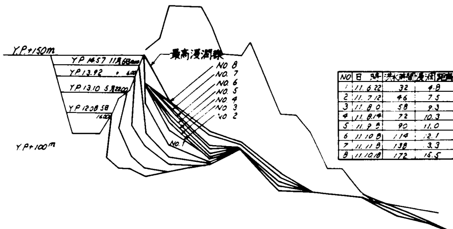
図-7.28 江戸川堤防の実験結果
