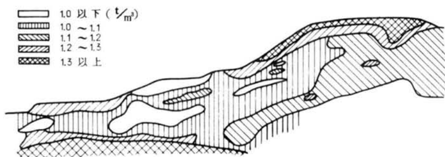
図一 7.5 降雨実験前の乾燥密度
