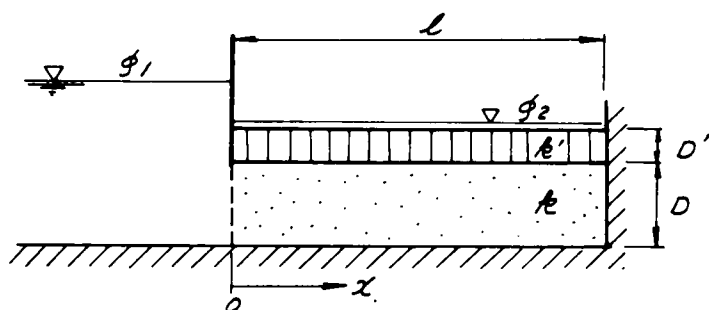
図-5.3 浸透条件 (a-ii)
