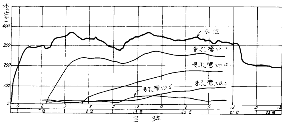
図-7.23 水位変化の測定結果
