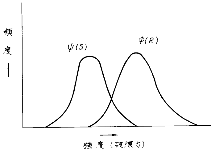
図-9.2 破壊の確率
