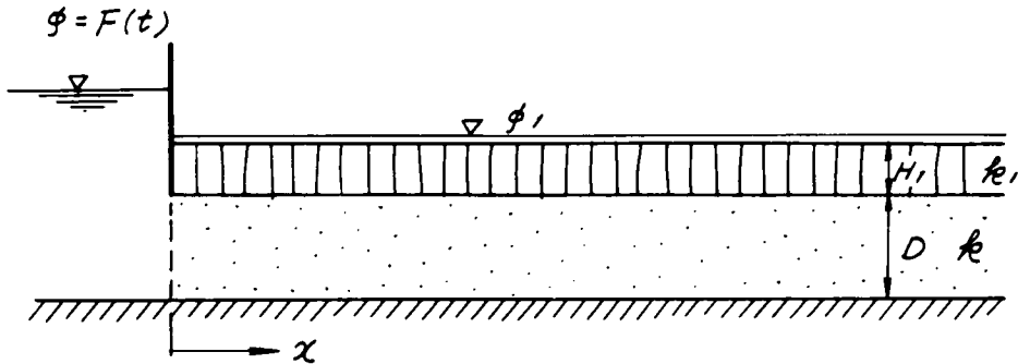
図-5.17 浸透条件 (2) IV)
