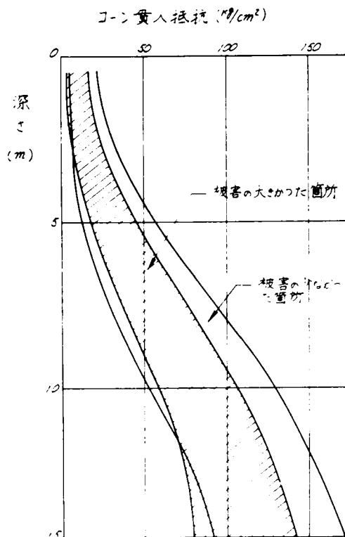
図-2.1.1 被害の大きかった箇所と少なかった箇所のコーン貫入抵抗の比較
