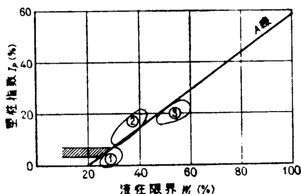
図- 3.4 塑性図による土質分類
