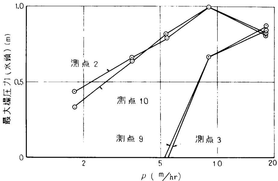
図-8.15 P と最大揚圧力の関係
