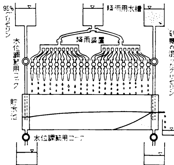
図-6.3.3 粘性流模型実験装置
