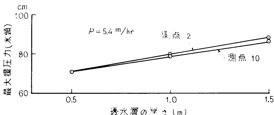
図一 8.1 6 透水層の厚さと最大揚圧力の関係
