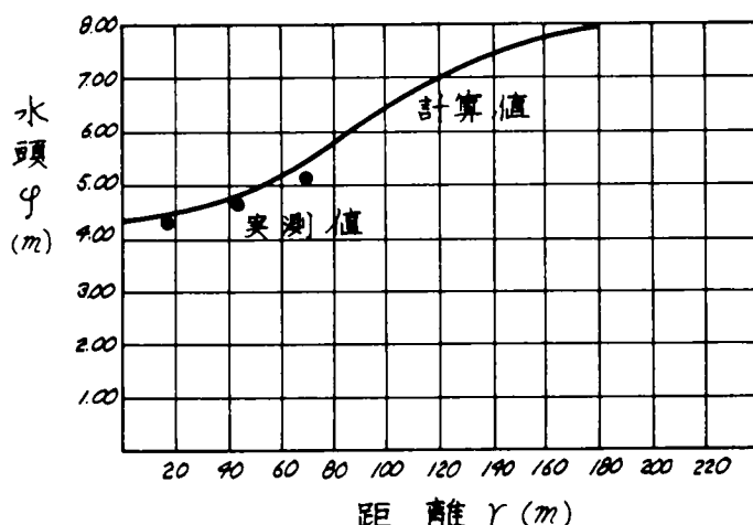
図 - 5.28 計算値と実測水頭の比較
