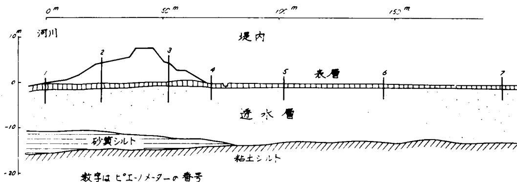
図-5.2.1 長良川堤防および基礎地盤(1.6 km付近)
