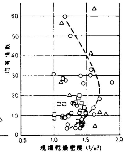
図-3.6 均等係数と乾燥密度の関係
