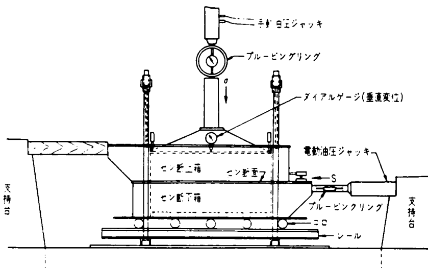
図-4.1.1 大型直接せん断試験機
