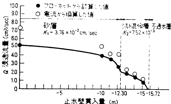
図-6.8 止水壁貫入量と浸透流量の関係
