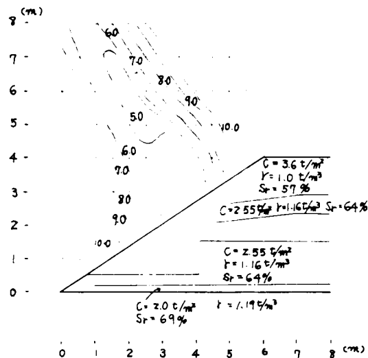
a 実験前の盛土の安定計算結果
