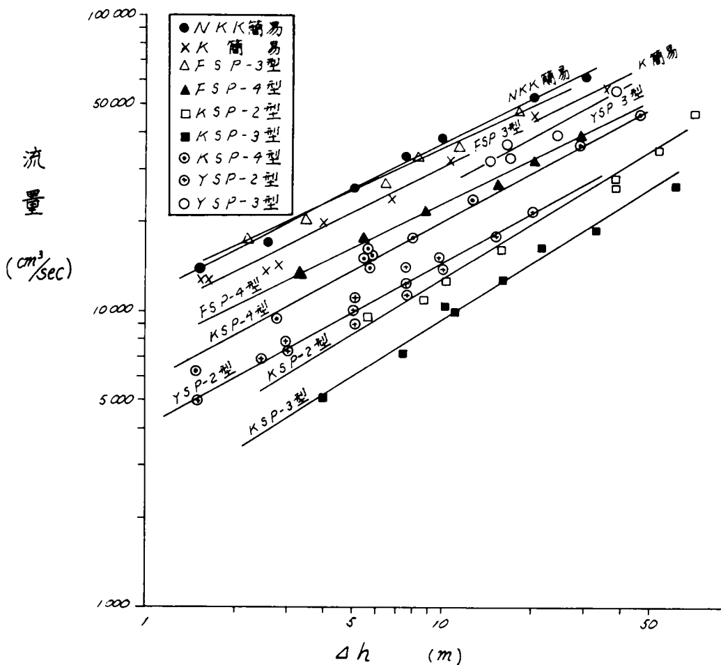
図一6.15 矢板のみの場合の矢板継手からの漏水流量
