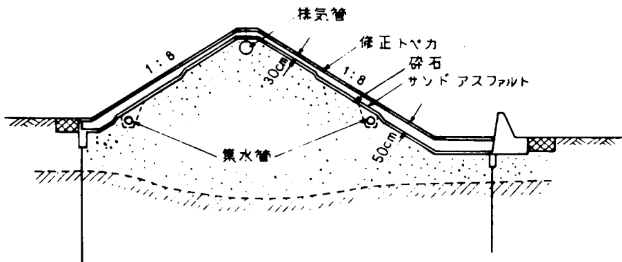
図-8.5 越流堤の構造
