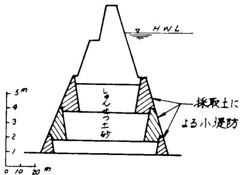
図- 7. 25 堤防の構造
