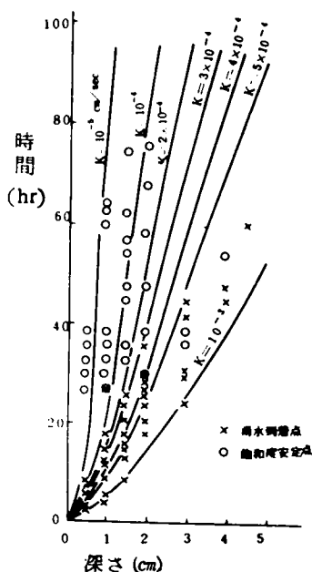
図-7.9 浸潤前線の深さと時間の関係
