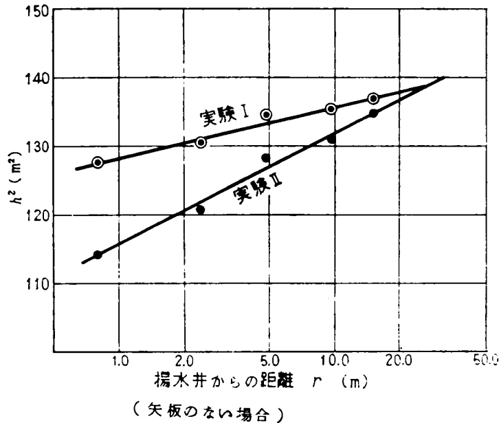
図-6.2.4 観測井の水位と観測井までの距離
