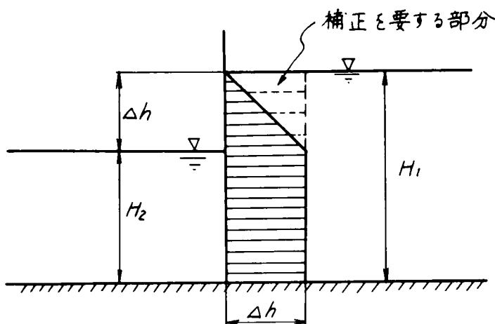
図-6.14 漏水流量の補正
