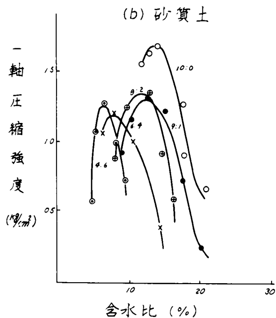
図-4.7 締固めた土のれき含有率と一軸圧縮強度 および含水比の関係
