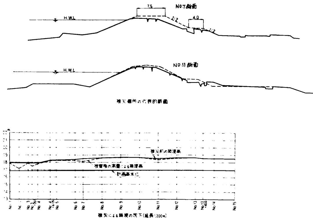
図-2.7 信濃川右岸真野代新田の堤防被害
