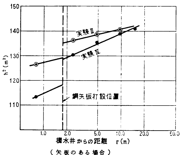
図－6.25 観測井の水位と観測井までの距離
