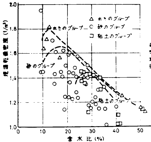
図-3.5 乾燥密度と含水比の関係
