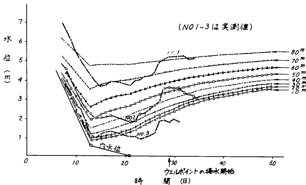
図- 5.29 水頭の実測値ならびに計算値
