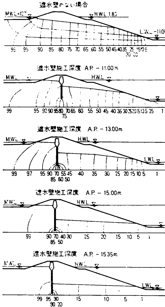
図-6.7 実験によって求めた等ポテンシャル線
