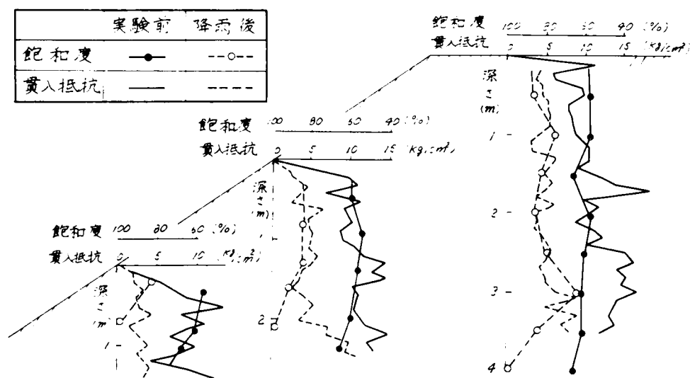
図-7.34 堤体内の飽和度とコーン貫入抵抗
