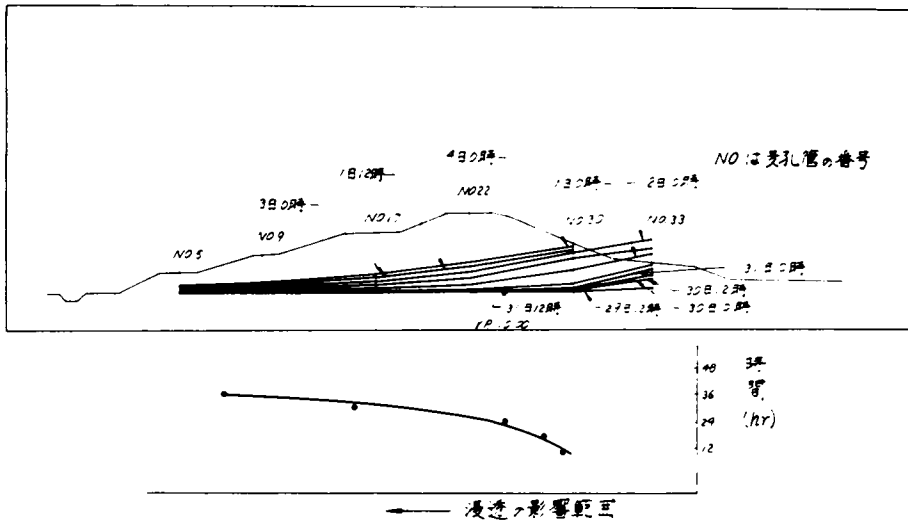
図-7.27 堤防の浸潤線の変化
