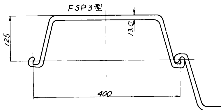
図-6.10 矢板の断面図
