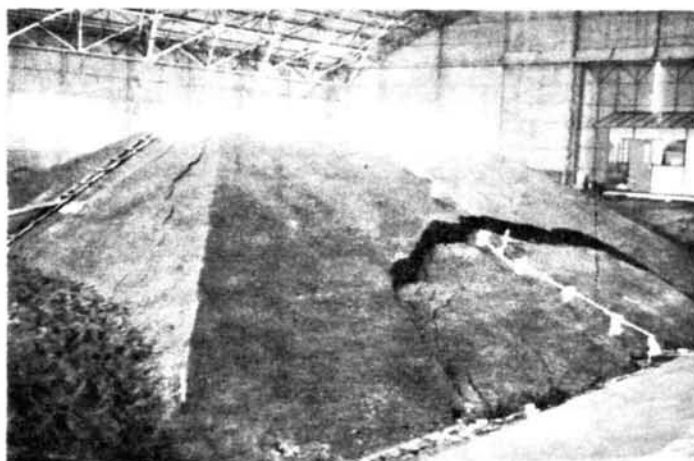
写真-7.1 実験堤防の斜面崩壊
