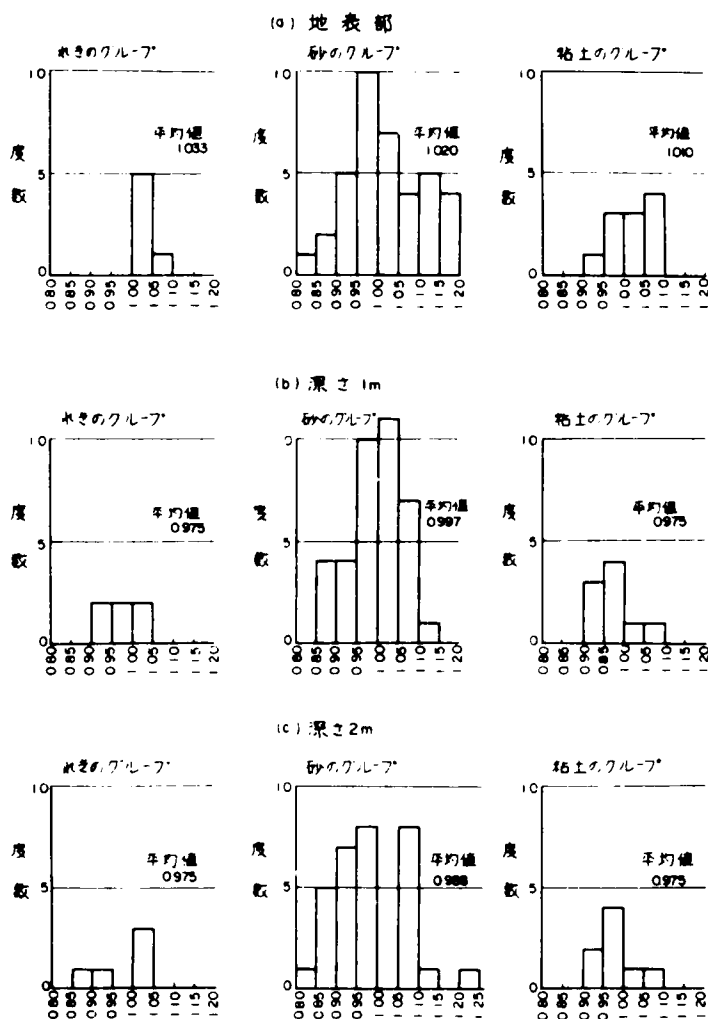
図- 3.1 4 乾燥密度のばらつき
