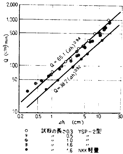
(a) 川砂に埋め込んだ鋼矢板
