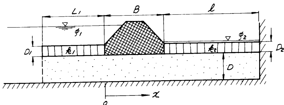
図-5.13 浸透条件 (a-VI)
