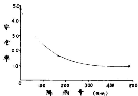
降雨量と安全率の関係
