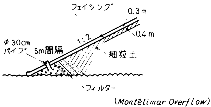
図-8.2.1 排水工の例
