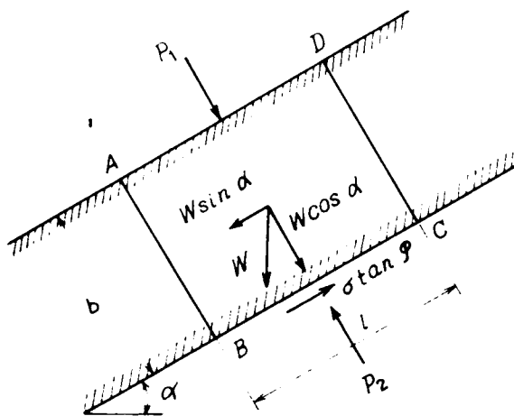
図-8.6 フェイシングの微少部分の釣合
