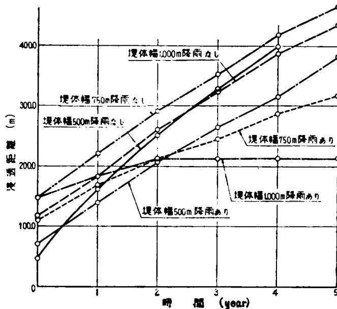
図-6.35 堤体内の塩水くさび先端の移動
