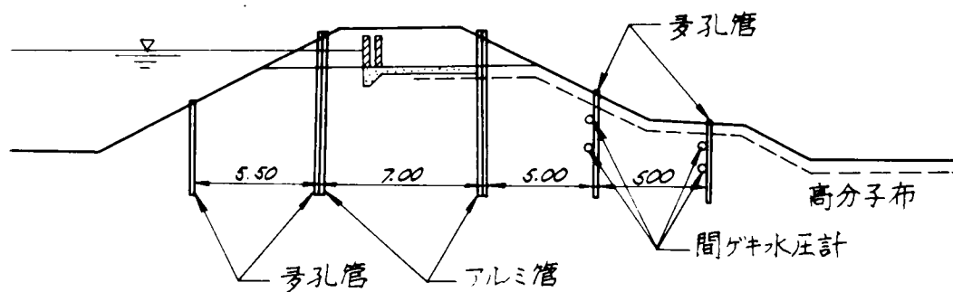
図－9.11 計器類埋設箇所
