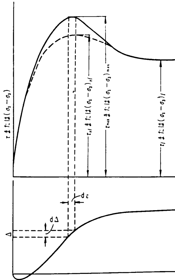
図-4.15 砂のせん断応力-ひずみ応力
