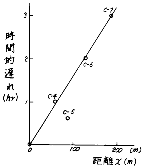
図-5.24 ピークの時間の遅れ
