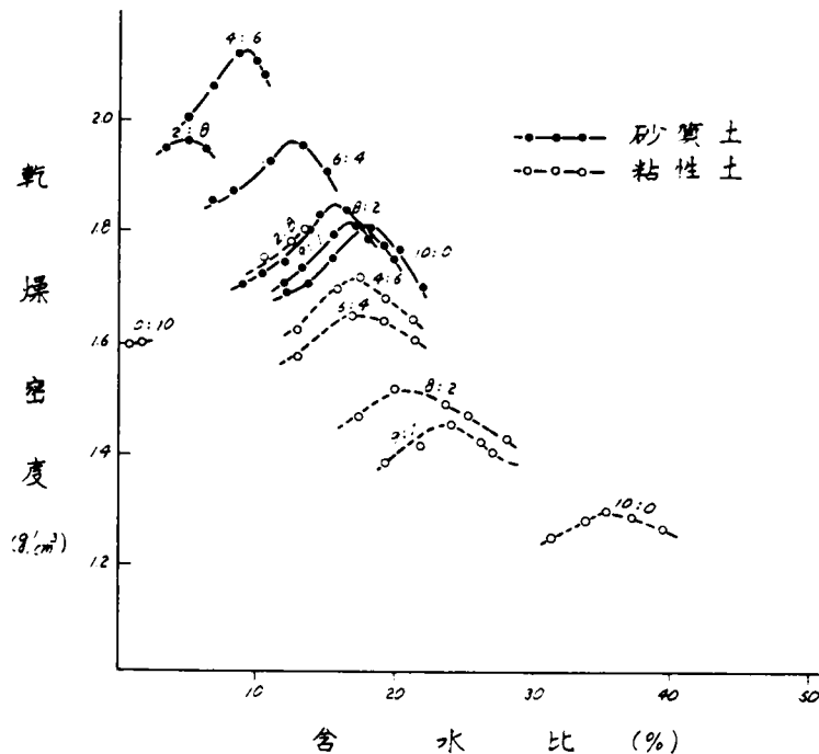
図-4.3 各試料の突固め曲線
