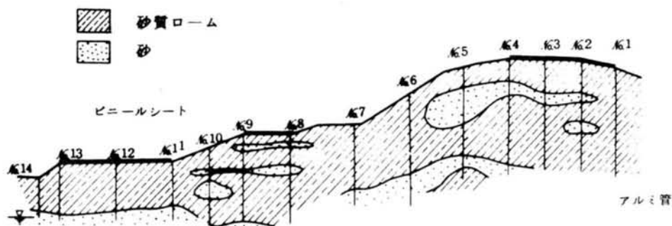
図-7.4 実験堤防の土質分布
