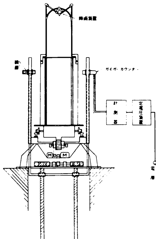
図-7.15 小型模型実験装置
