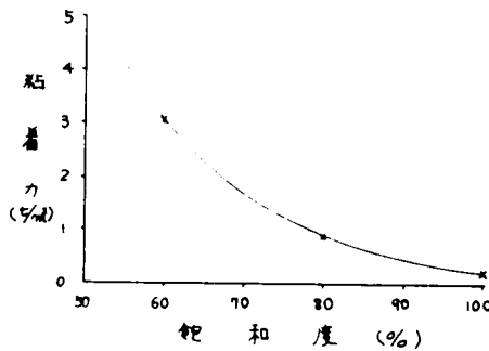
図-7.3.6 飽和度と粘着力との関係
