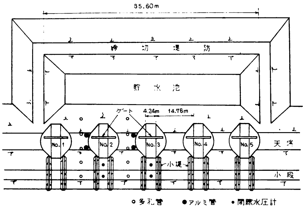
図-9.9 実験堤防の平面図
