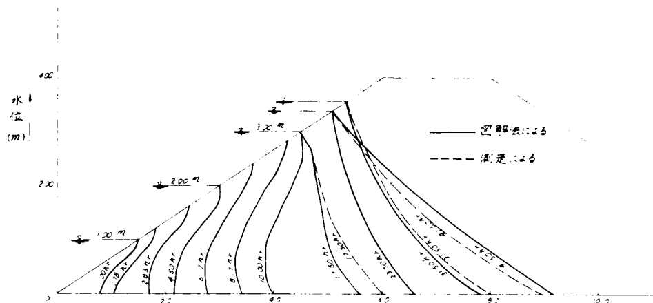
図-7.2.1 図解法による結果と実測値の比較
