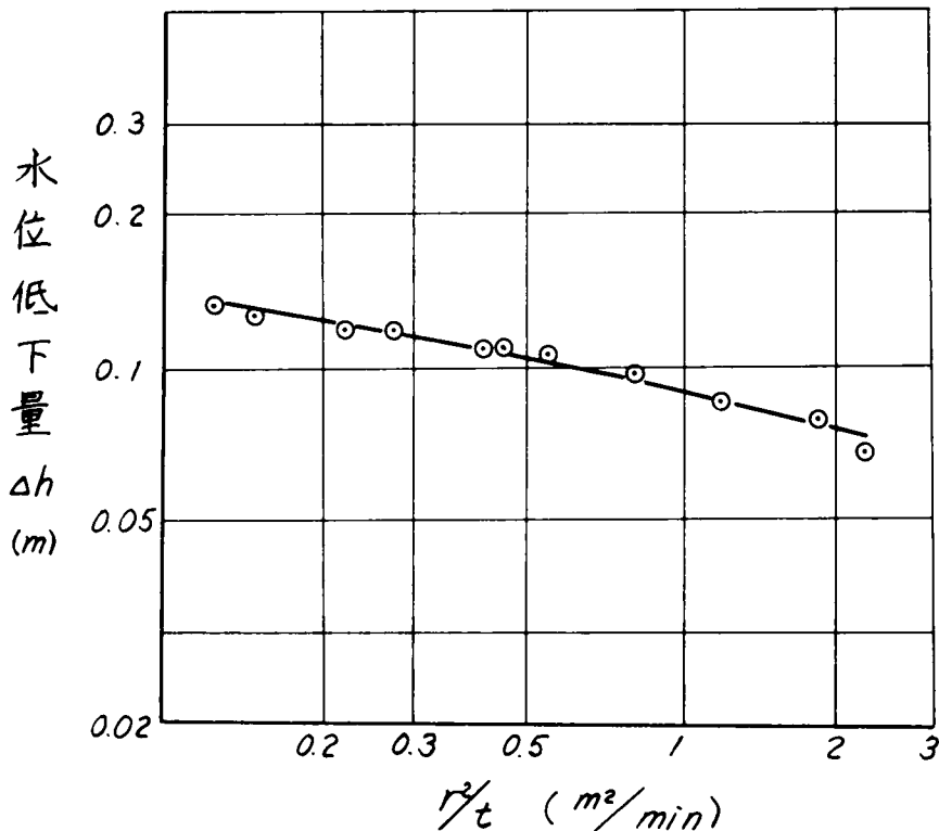
図-5.3.1 揚水試験の結果の一部
