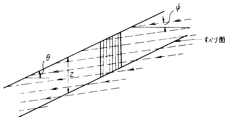
図-2.3 浸透水のあるのり面
