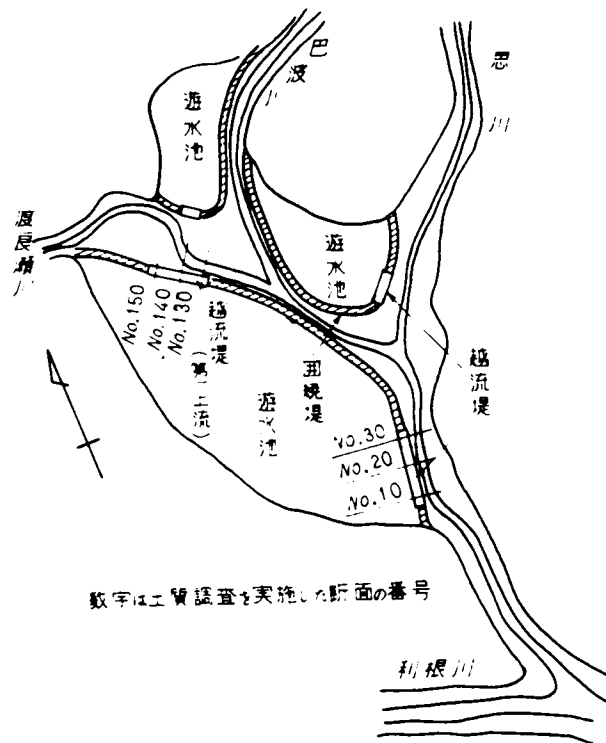
図－8.1 渡良瀬川越流堤築造箇所平面図
