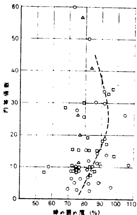
図-3.1.0 均等係数と締め固め度の関係
