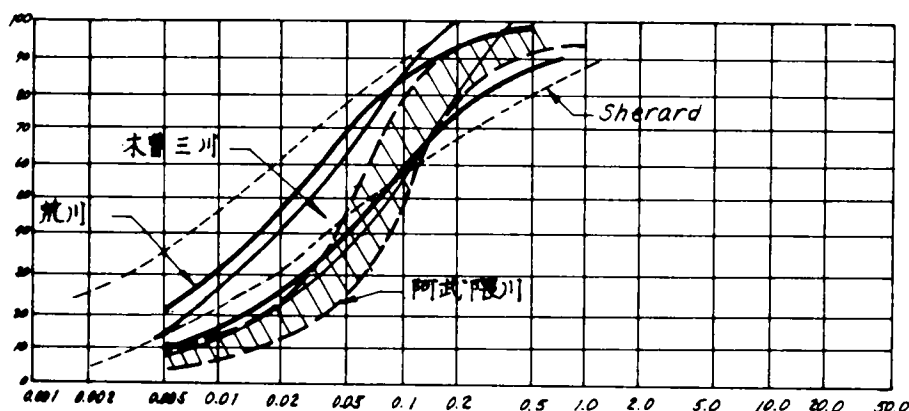
図-2.2 のりすべりを起こした堤体材料の粒度曲線の範囲
