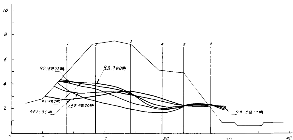
図-7.31 阿武隈川堤防の浸潤線の変化
