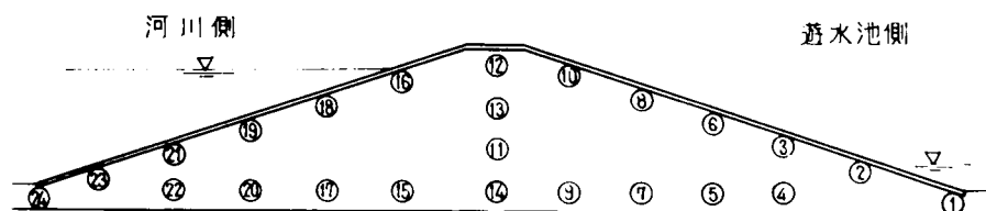
図-8.11 間げき圧測定装置設置箇所
