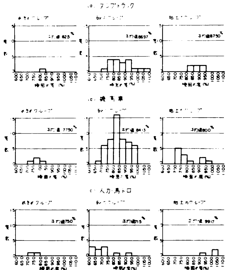
図- 3.15 施工法による締固め度のばらつき
