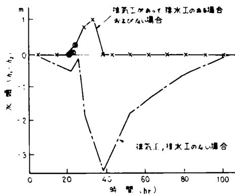
図-8.18 天端のフェイシングに作用する水頭
