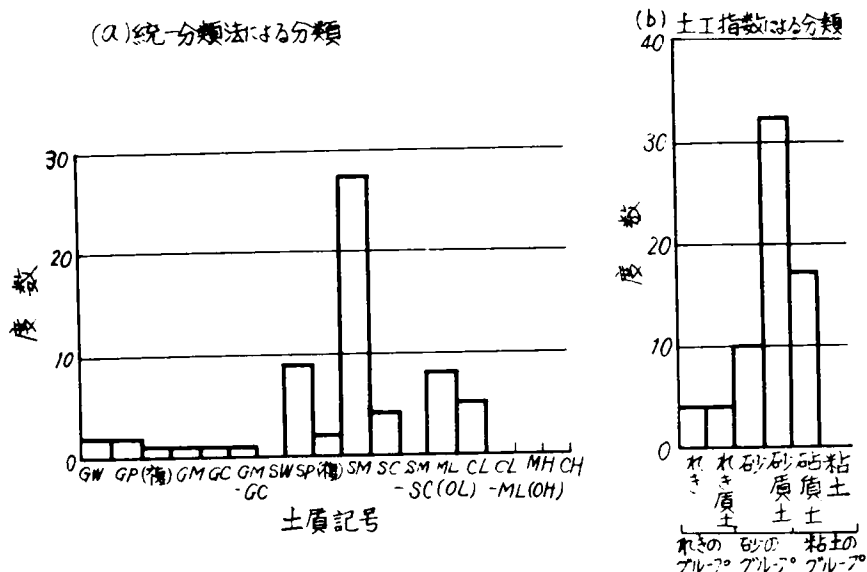
図- 3. 2 堤体材料の分類
