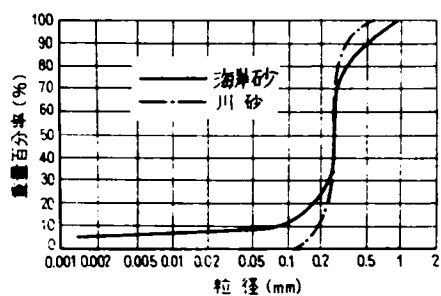
図-6.11 粒度曲線
