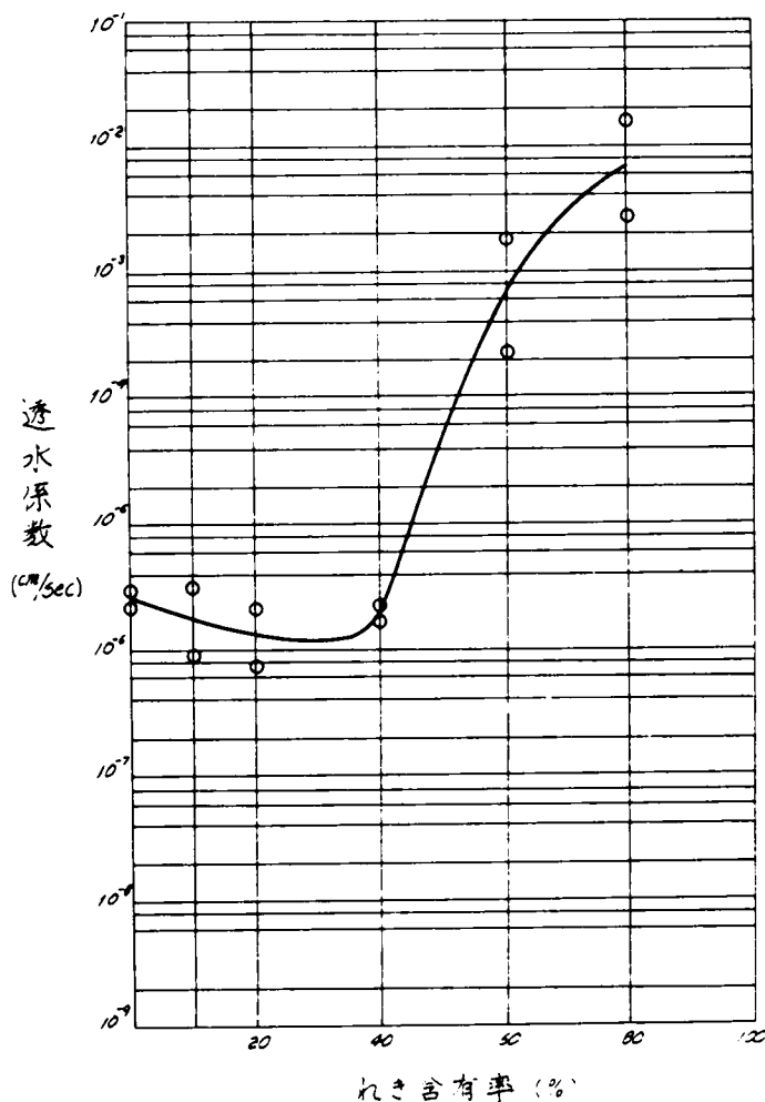
図-4.8 れき含有率と透水係数
