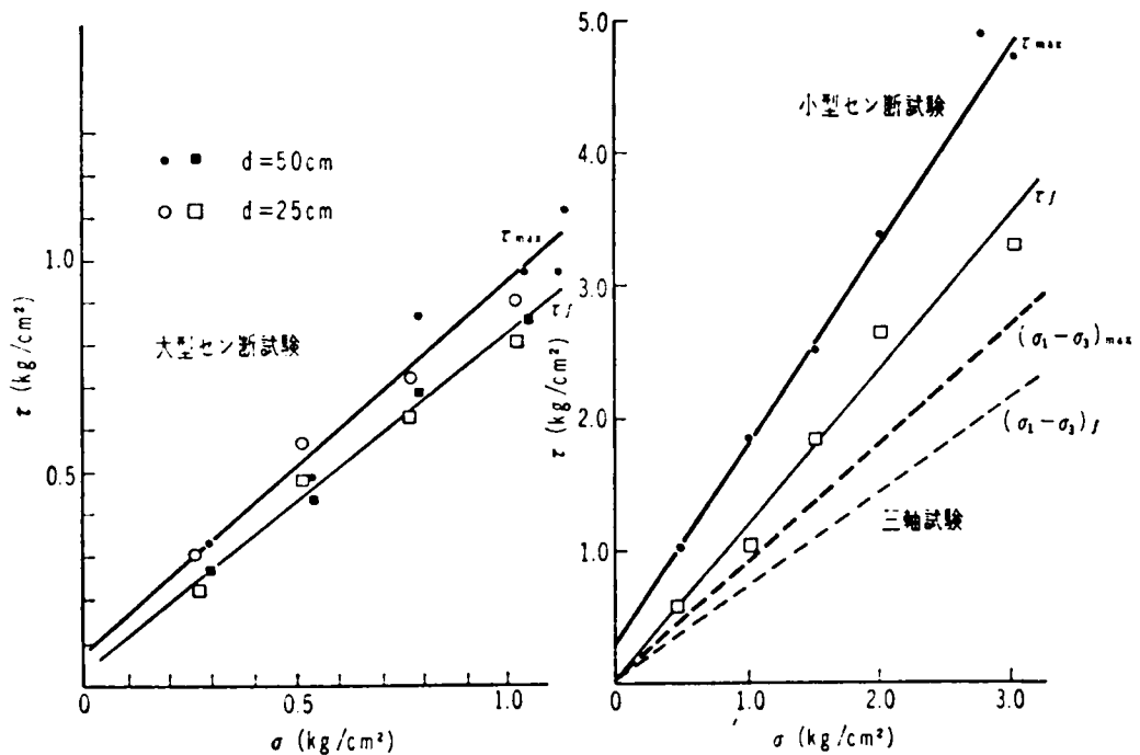
図一 4.1.4 各種試験機による試験結果
