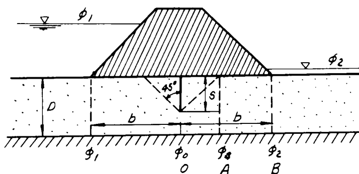
図-6.1 簡単な基礎地盤の浸透
