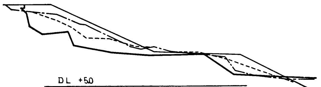
図 - 9.12 実験堤防の洗掘状況
