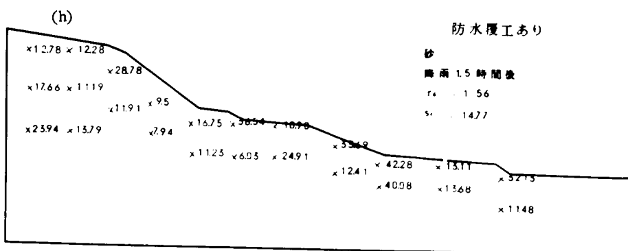
図-7.16 小型模型実験によつて求めた飽和度(%)
