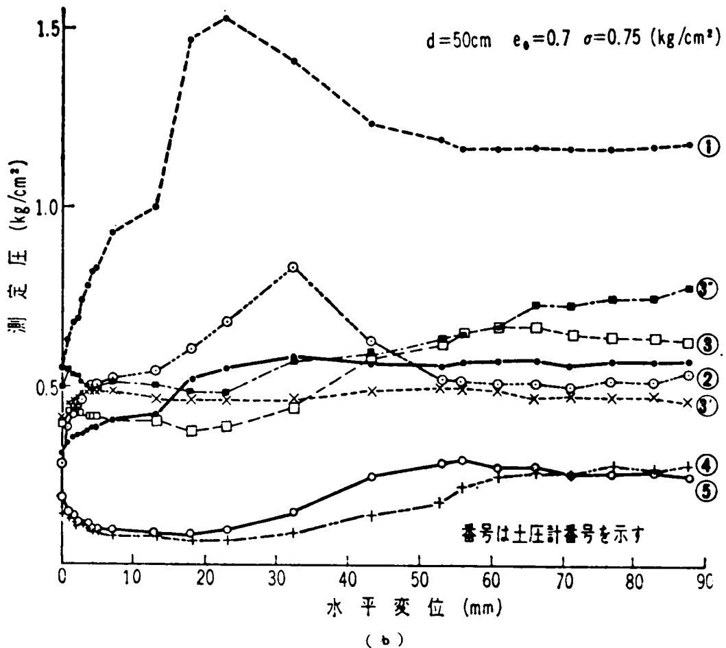
図- 4.17 セン断箱底面の圧力分布 (b)
