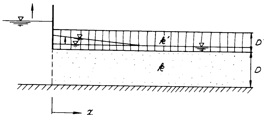
図-5.16 浸透条件 (2) i)
