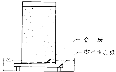
図-7.10 毛管水頭と飽和度の関係を調べる装置
