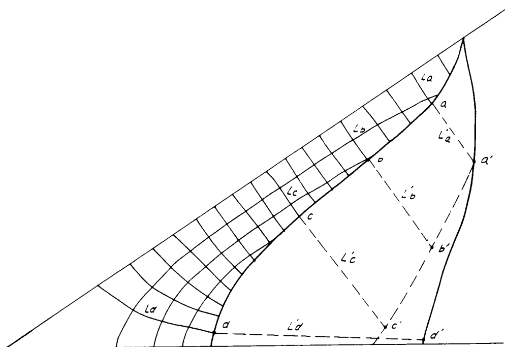
図－7.19 水位が瞬間的に上昇したときの図解法
