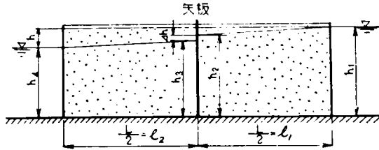
図-6.20 透水層内の浸透
