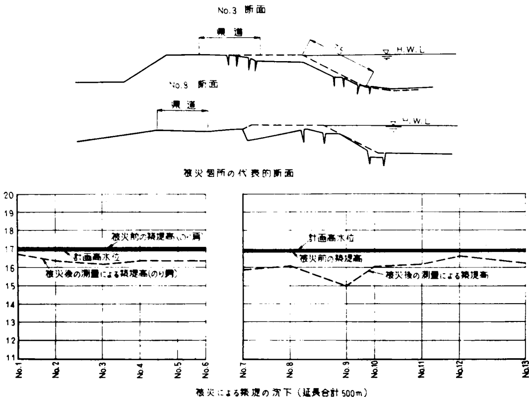
図-2.8 信濃川左岸町軽井堤防の被害
