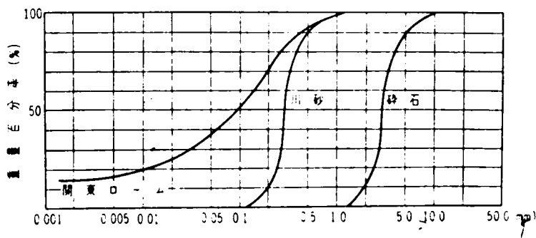
図一 4.1 3 試料の粒度曲線
