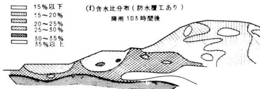
図一 7.6 堤体内の含水比の変化
