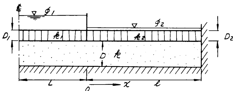
図-5.5 浸透条件 (a-IV)
