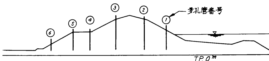
図-7.29 堤防断面ならびに多孔管設置位置
