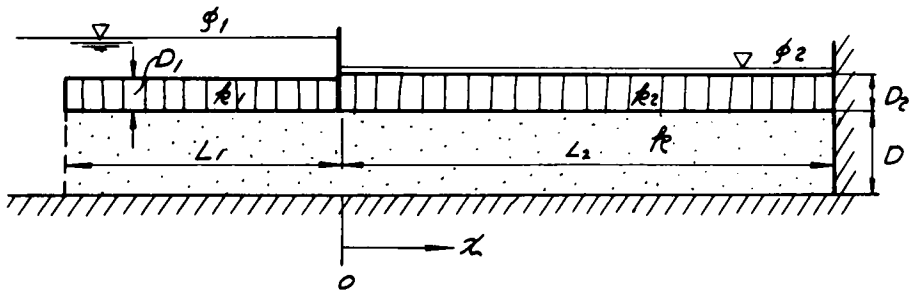
図-5.7 浸透条件 (a-VI)
