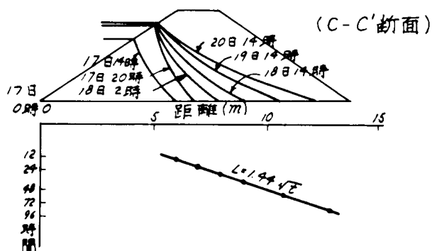
図-7.24 浸潤線の移動
