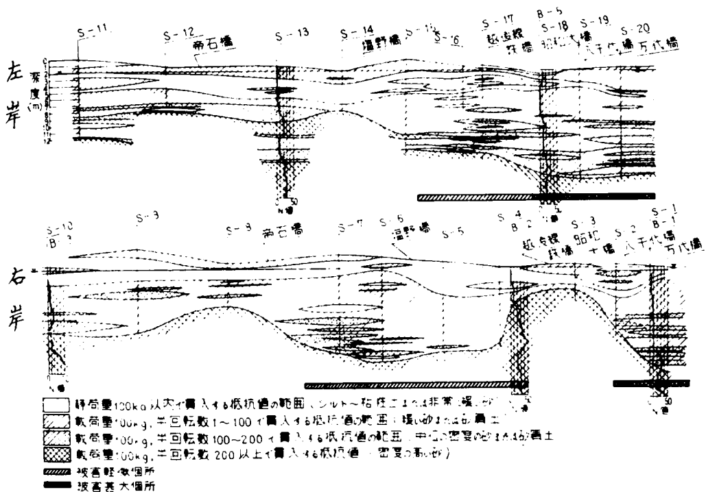
図-2.10 サウンディングによる地盤の抵抗と被害の程度
