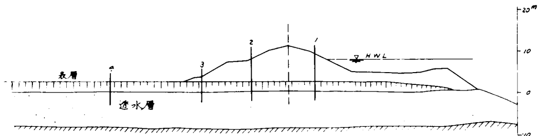
図-5.20 阿武隈川堤防および基礎地盤(寺島地区) 縦横1:1
