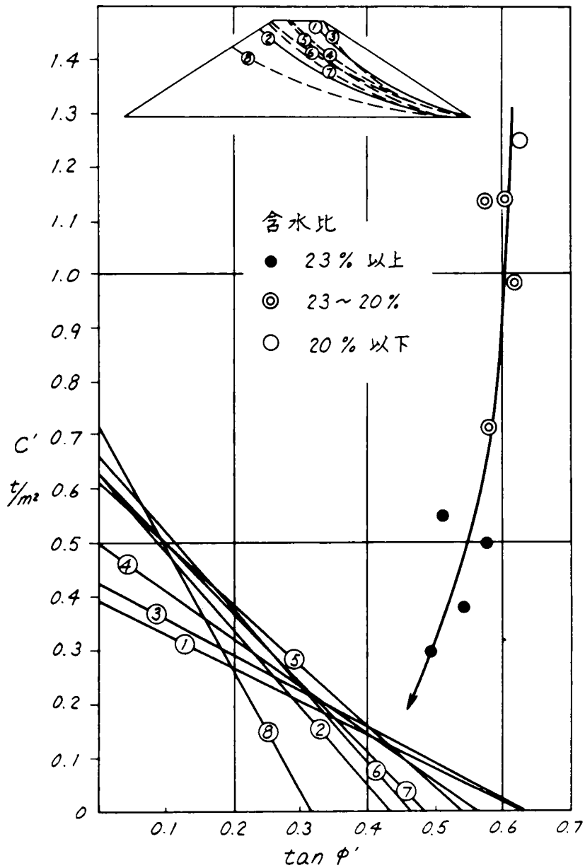
図-7.35 安定計算の結果とせん断試験の結果
