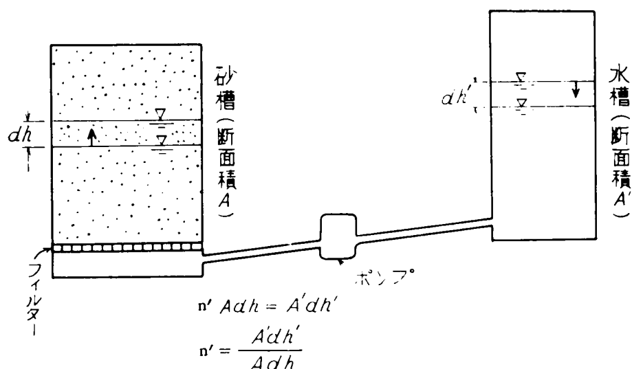
図-8.8 有効間げき率の測定装置の原理
