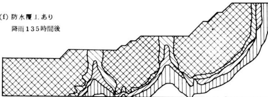
図-7.14 計算による堤体内の飽和度の変化
