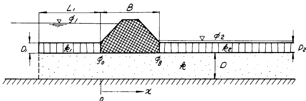
図-5.12 浸透条件 (a-V)
