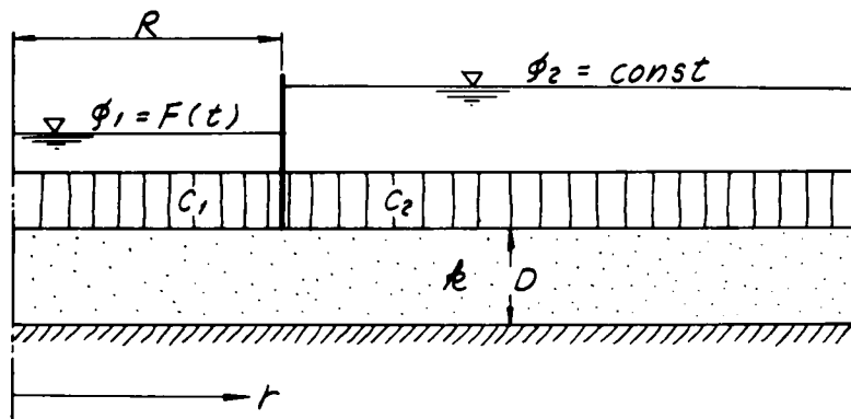
図-5.19 浸透条件(円形の縮切堤の場合)
