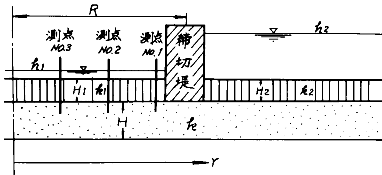
図-5.27 浸透条件ならびに水頭の観測位置
