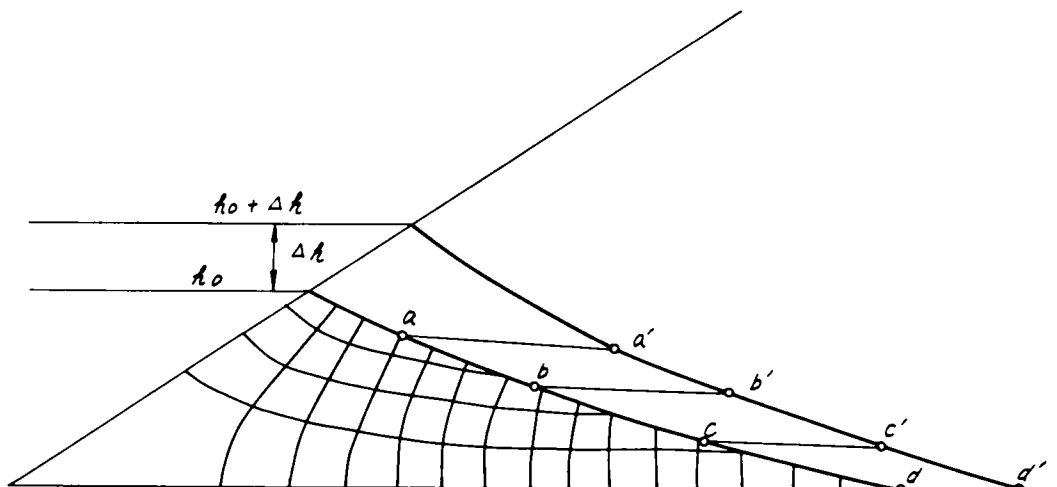
図-7.20 水位が変動するときの図解法
