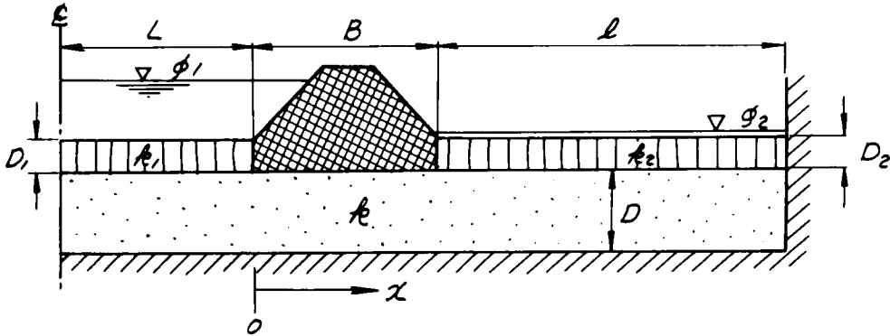
図-5.11 浸透条件 (b-iv)
