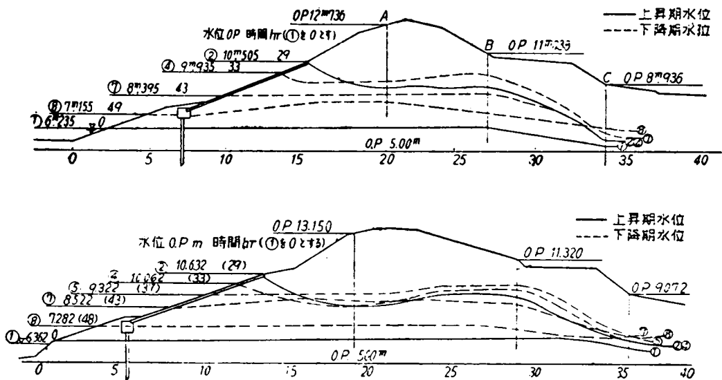
図-7.3.3 淀川堤防の浸潤線の変化
