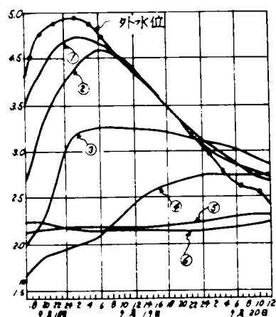
図-7.30 洪水時の水位変化
