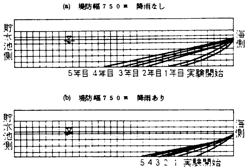
図-6.3.4 塩水くさびの移動
