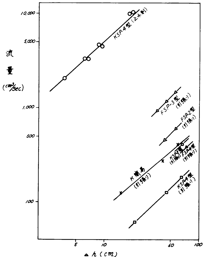
図-6.16 止水剤と引張りを加えたときの矢板継手からの漏水
