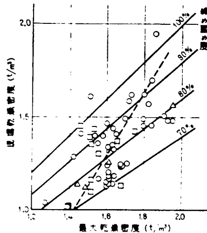
図-3.8 現場乾燥密度と最大乾燥密度の関係
