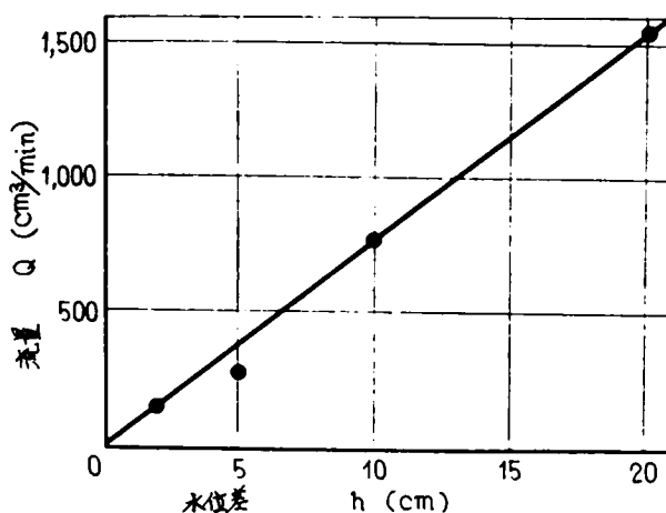
図-6.13 砂のみの透水実験における流量と水位差
