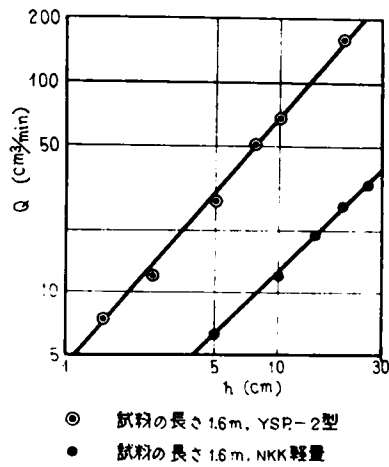
(b) 海岸砂に矢板が埋め込まれた場合の 水位差 h と流量 Q の関係
