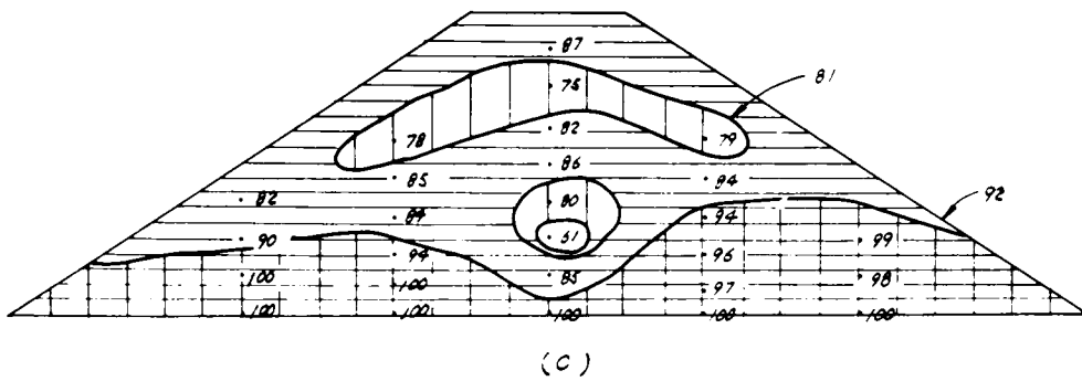
図-7.17 盛土内の飽和度の変化
