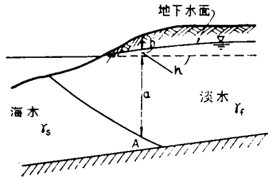
図-6.3.2 2流体の境界面
