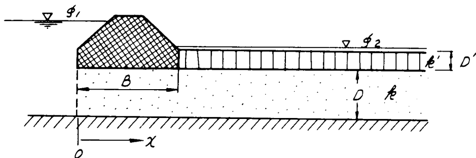
図-5.8 浸透条件 (b-i)
