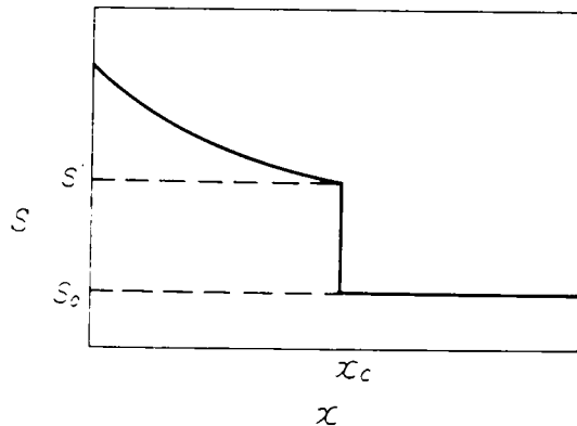
図-7.1 飽和度の分布
