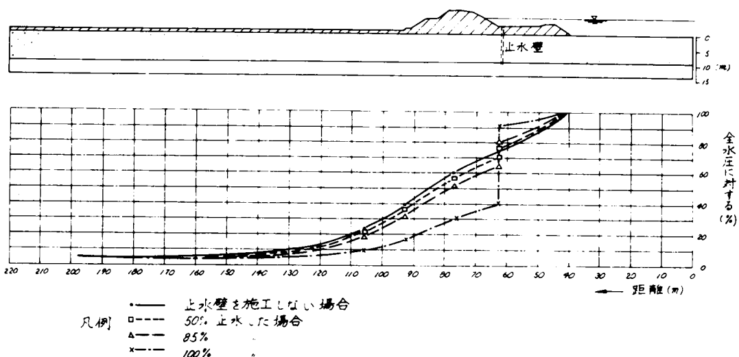
図-6.6 表層の下に働く水頭分布の比較
