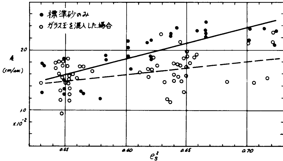
図-4.9 砂の間げき比 e_s と透水係数 k の関係
