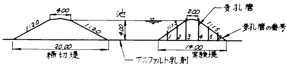
図-7.22 実験堤の断面
