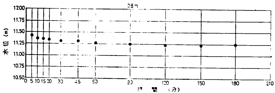
(a) 実験 I 鋼矢板のない場合
