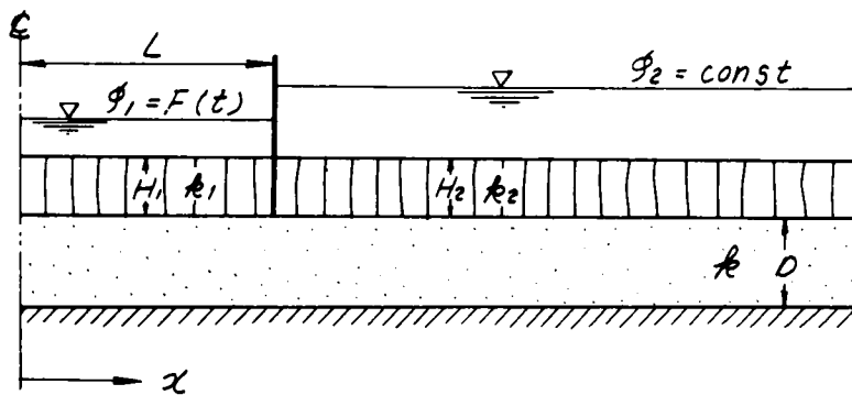
図-5.18 浸透条件(平行な締切堤の場合)
