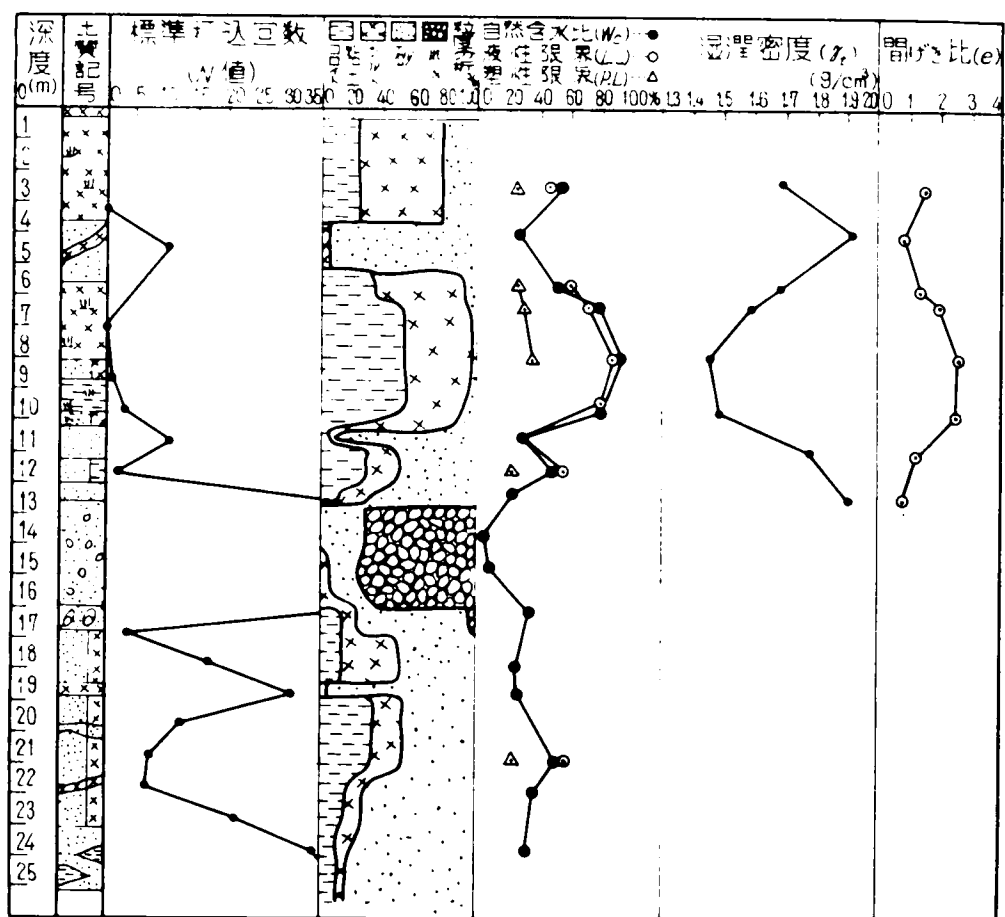
図- 8.3 渡良瀬越流堤築造地点の代表的ボーリング調査結果
