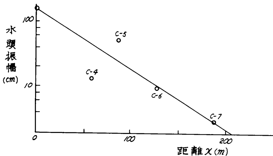
図-5.23 振幅と距離の関係
