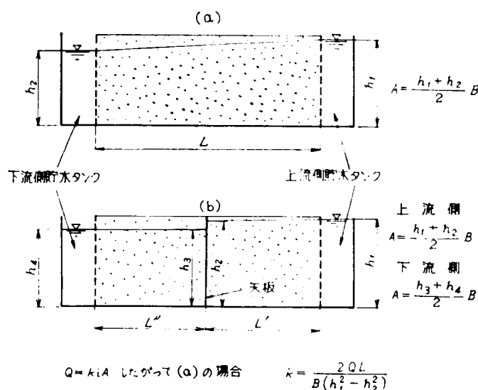
図-6.12 透水係数の算出
