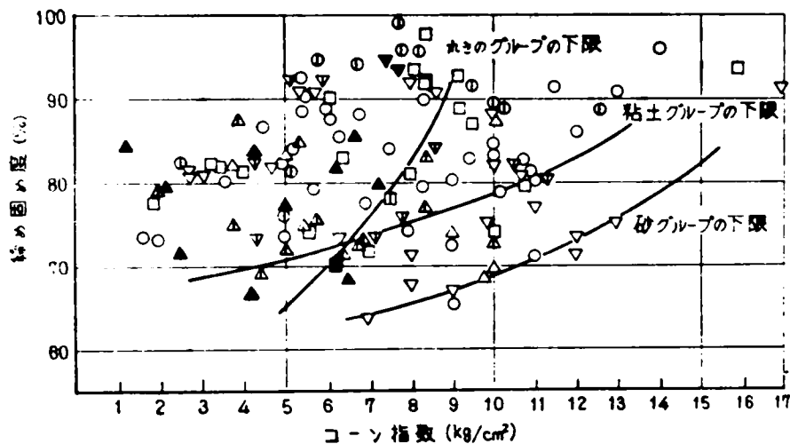
図-3.1.2 締固め度とコーン指数の関係
