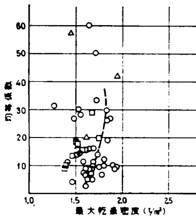
図-3.7 均等係数と最大乾燥密度
