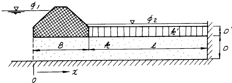
図-5.9 浸透条件 (b-ii)
