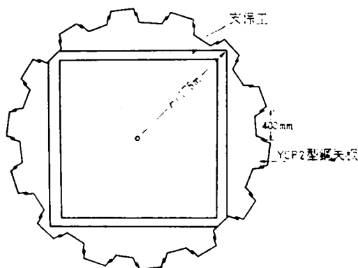
図-6.2.1 鋼矢板の配置
