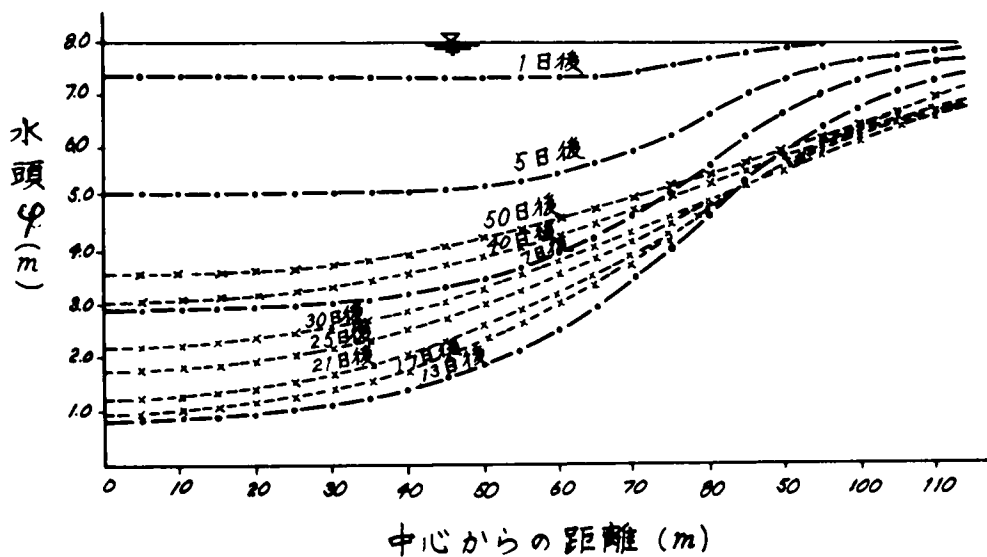
図- 5.30 透水層内の水頭分布
