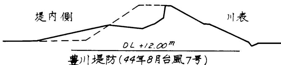
図－9.8 越流してかろうじて破堤をまぬがれた堤防の1例
