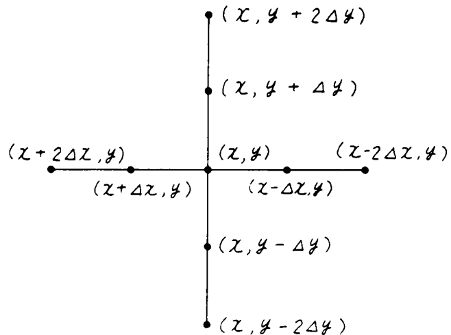
図-7.13 格子点の記号
