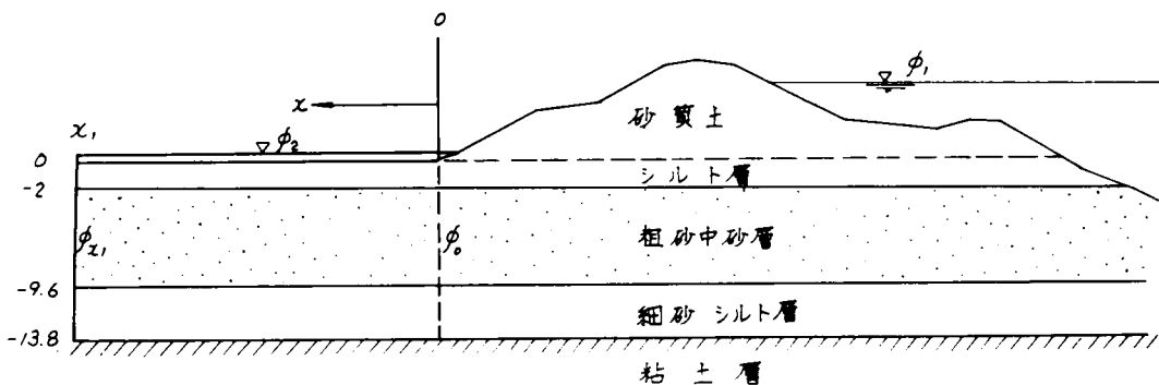
図-6.4 阿武隈川堤防の地盤構成
