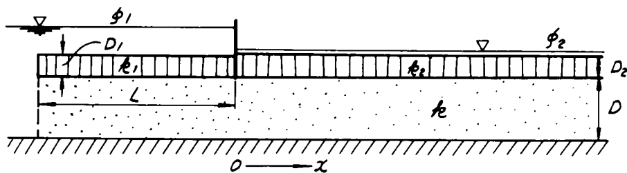
図-5.6 浸透条件 (a-V)
