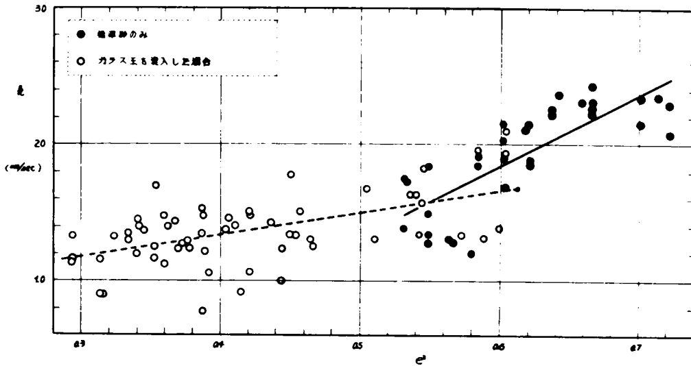
図－4.10 全体の平均間げき比 e と透水係数 k の関係
