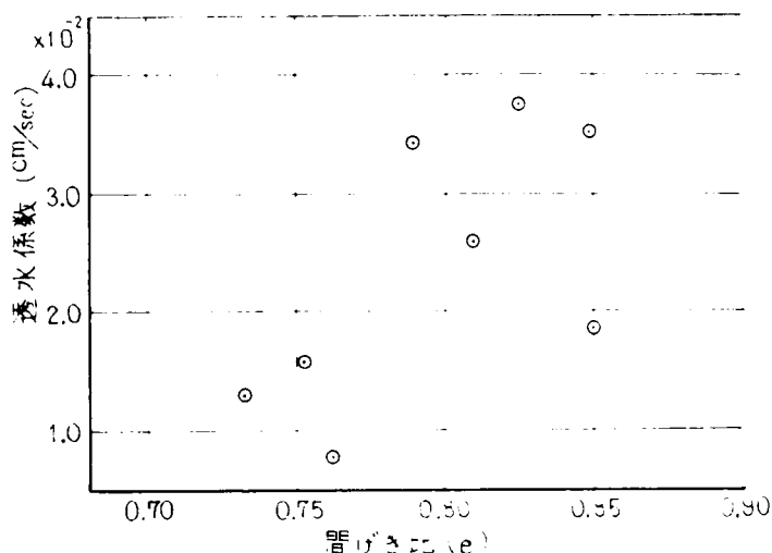
(a) 室内試験による透水試験
