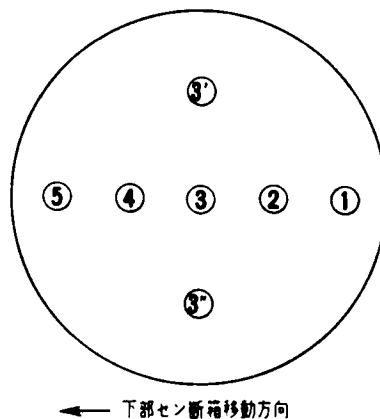
図-4.12 土圧計配置図
