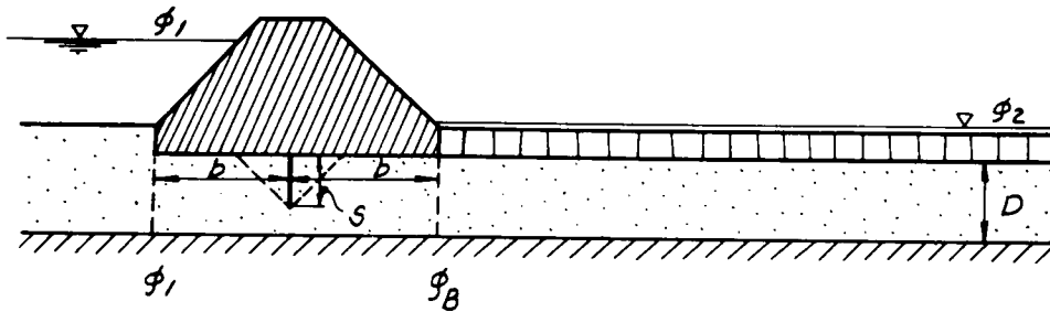
図-6.2 半透水性表層がある場合の浸透
