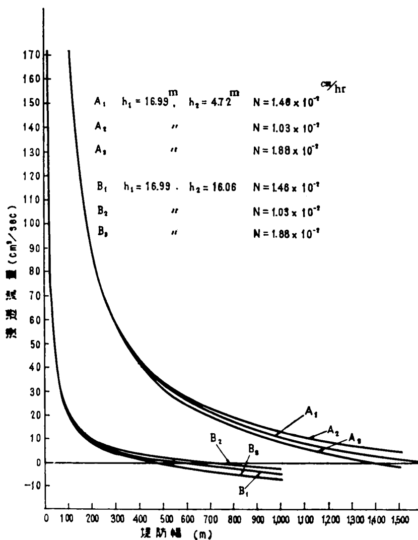
図-6.29 堤防幅と浸透流量の関係
