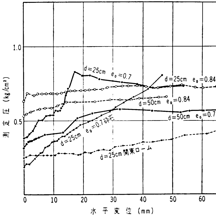
図-4.18 セン断箱底面の平均圧
