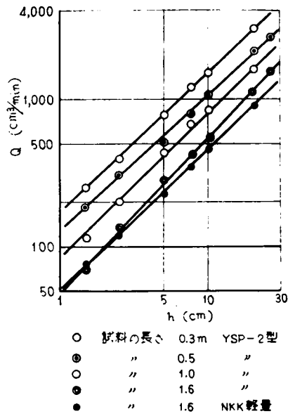
(a) 川砂に矢板が埋め込まれた場合の水位差 h と流量 Q
