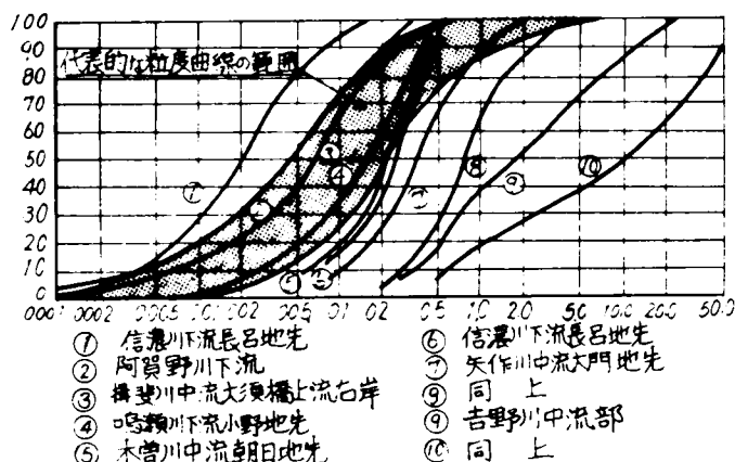
図- 3. 3 東北地方の河川堤防材料の代表的な粒度曲線の範囲と各地方の堤防の粒度曲線
