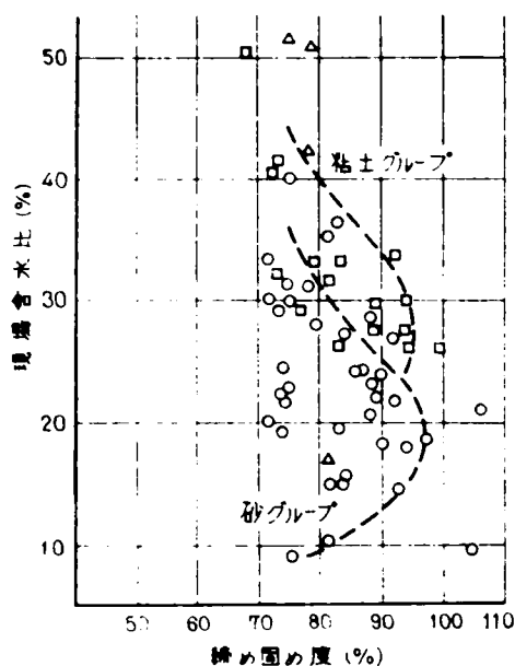
図- 3.9 現場含水比と締固め度の関係
