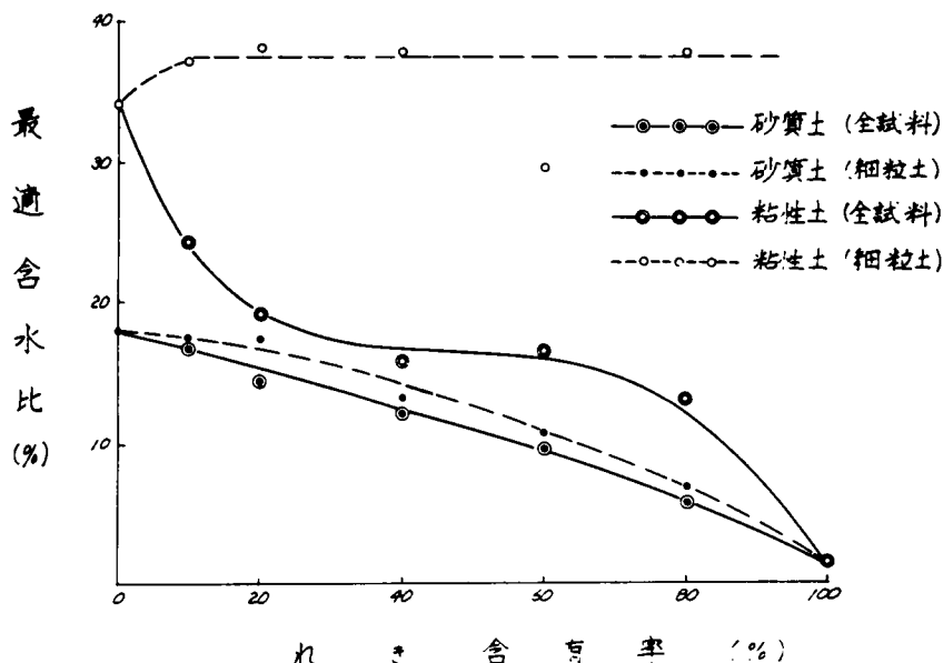
図-4.4 れき含有率と最適含水比の関係
