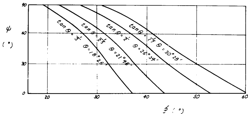
図 2.4 のり面の安定計算の例
