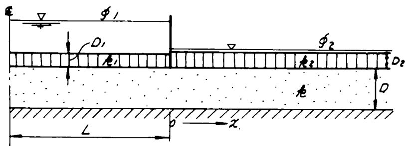
図-5.4 浸透条件 (a-iii)
