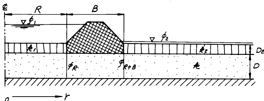
図-5.15 浸透条件 (c-ii)
