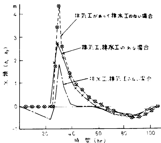
図-8.19 のり尻付近のフェイシングに作用する水頭
