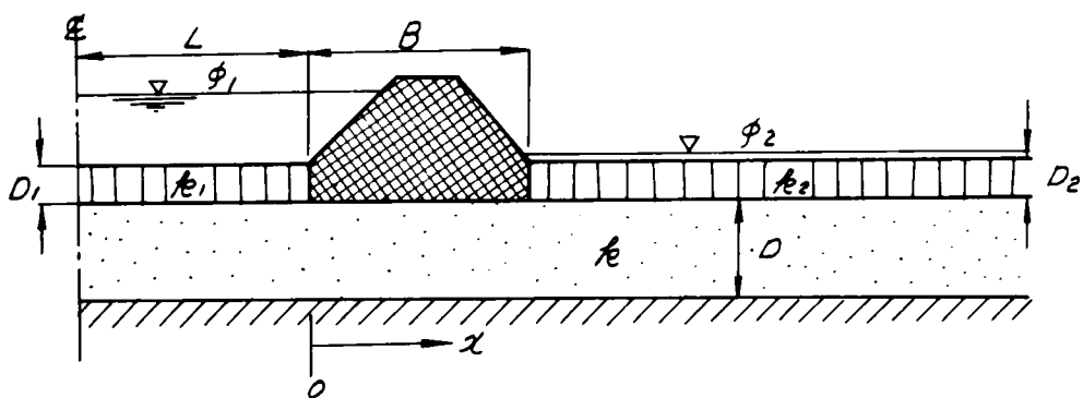
図-5.10 浸透条件 (b-III)
