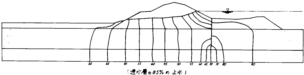
図-6.5 実験で求めた等ポテンシャル線の1例
