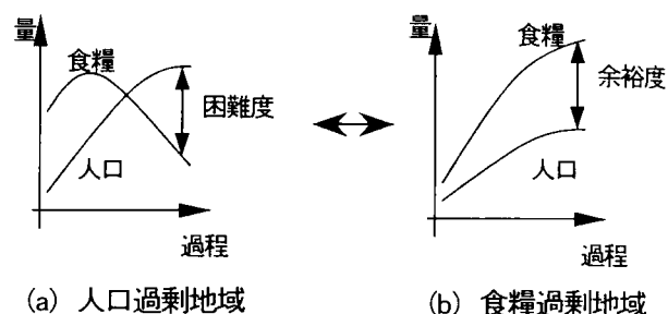
図6.23 現代の推移
