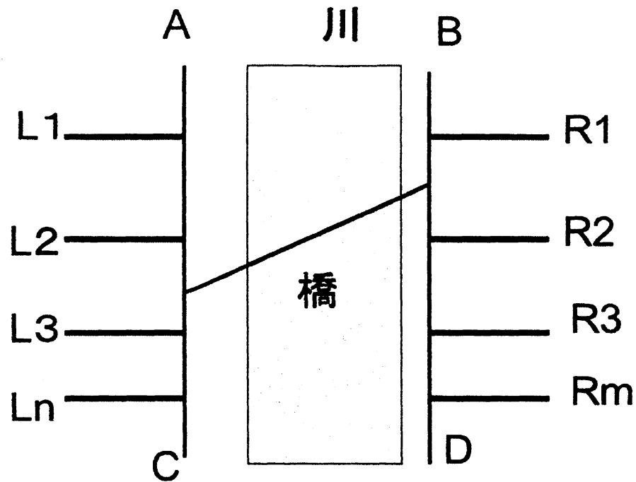
Figure 4.1: 川をはさんで、左・右の道路の交通量は、ファジィ数 A, L_1, L_2, \dots, L_n, C; B, R_1, R_2, \dots, R_m, D で与えられるモデルである。
