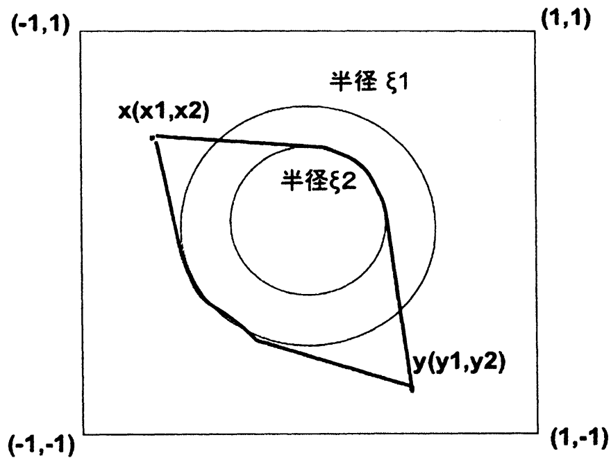
Figure 5.1: 障害物の半径は \xi_1, \xi_2 \in [R_1(\alpha), R_2(\alpha)] , \alpha は帰属度、とする。2点 x, y を自由にとり、帰属度 0 < \alpha \leq 1 に応じて、半径 \xi_i \in [R_1(\alpha), R_2(\alpha)] を決める。自由スペース内の x-y 間最短パスを見出すためには、いくつかの計算の可能性が生じる。
