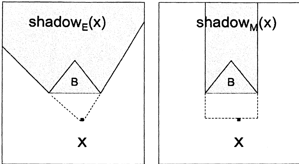
Figure 2.1: E(= \|\cdot\|_1) ノルムによる影 (左図) と, M(= \|\cdot\|_\infty) ノルムによる影 (右図) とは異なる.
