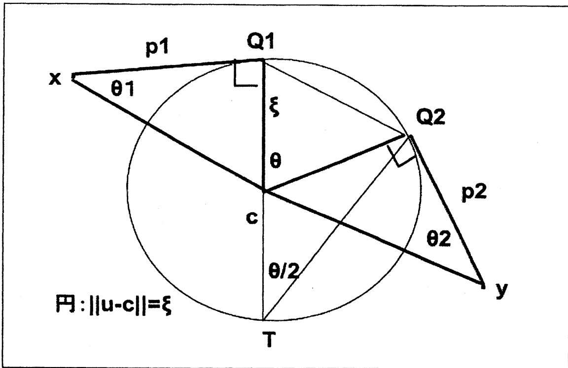
Figure 3.2: 障害物の境界は中心 c \in \mathbb{R}^2 , 半径 \xi, \xi \geq 1 で, 点 x, y とは点 Q_1, Q_2 で接する. ベクトル c-x と Q_1-x , Q_2-y と c-y , Q_1-c と Q_2-c のなす角を各々 \theta_1, \theta_2, \theta とする. なお反時計方向を正とする. T を線分 Q_1c を c の方向に延ばした直線と境界 \partial B_{\xi,c} の交点とする.
