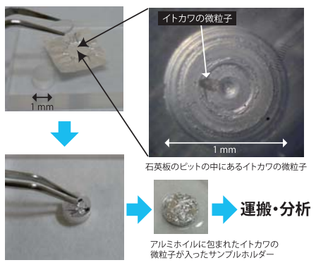
図 イトカワの微粒子を運搬する方法 直径9ミリの石英板に設けた直径1ミリのピットに粒子を格納し、ピットなしの石英板で挟んで、アルミホイルに包んで運搬します。中性子照射やその後の分析もこのまま行われます。 海老原克ら、Science 333, 1119(2011) Supporting Online Materialより抜粋
