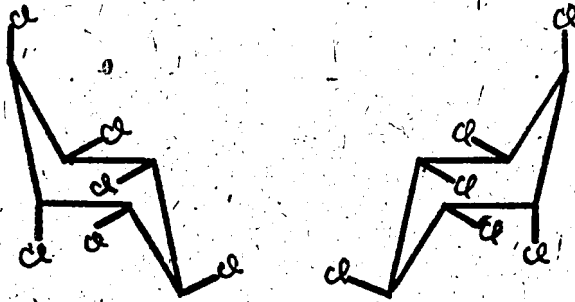
1, 2, 4 椅子型鏡面異性体 ( \alpha ?)
