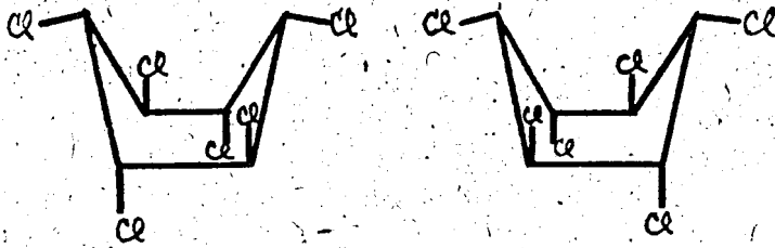
舟型鏡面異性体 ( \epsilon )
