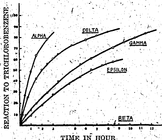
第 3 圖 BHC 異性体の脱鹽酸反應 (0.1 N methanol 性曹達, 0°C)
