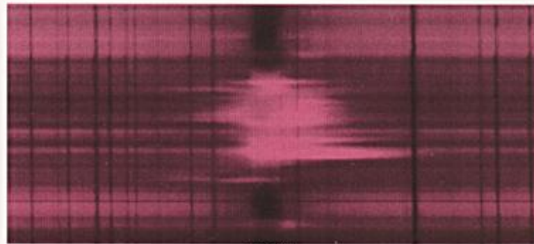
H \alpha 線
