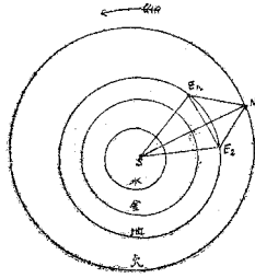
第四圖 一週して再び元のM點に來た時は地球はまだ元のE 1 に來らずしてE 2 に在る筈である。然らばE 2 に於ける火星の離角S E 1 M、S E 2 Mは觀測によつて知ることが出来る。又角はE 1 S E 2 地球が四十三日五八にて廻轉する角度であつて大凡四十三度である。
