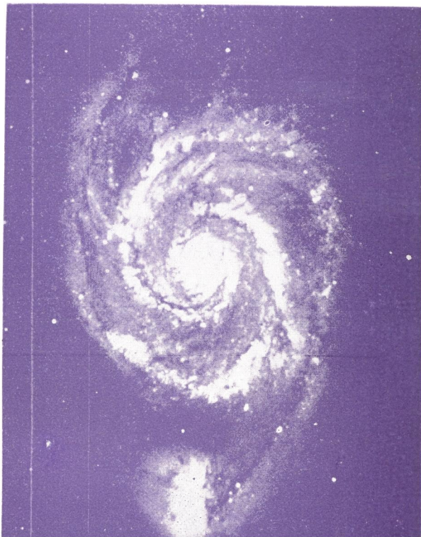
獵犬座の渦巻き「M五十一」
