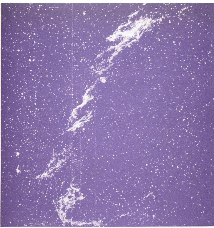
白鳥座のガス星霧
