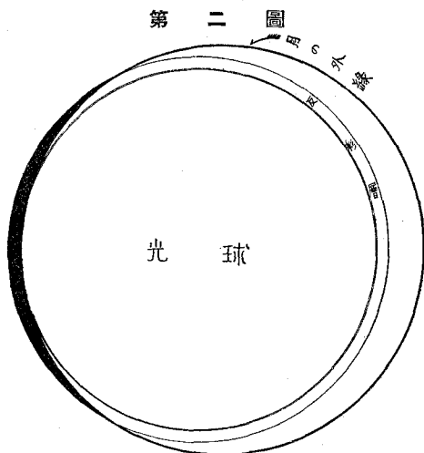
内光スペクトル撮影時に於ける太陽と月の位置左方黒い三日月形の部分が内光スペクトルとなつて現はれる。
