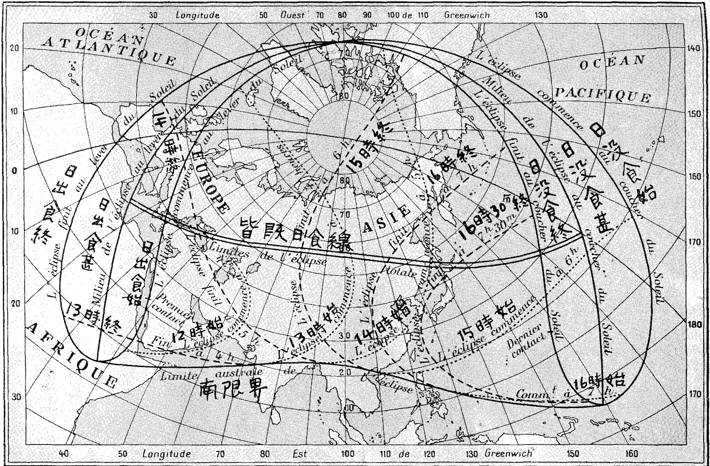
1936年六月19日皆既日食圖 (佛曆より)
