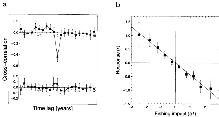
図 2: 漁獲に対する線形応答。(a) \Delta f と r (上) および \Delta f と \Delta \xi (下) との相関関数。 38 セットの時系列の平均値と 95% 信頼区間を示す。(b) 応答関数。 ICES データの個体群成長率 r を漁獲変動 \Delta f の各ビンで平均した値と 95% 信頼区間を示す ( x, y 軸は各個体群の \sigma_{\Delta f} および \sigma_r でスケールしてある)。 実線の傾きは時差 \Delta t = 0 の相関係数 (図 a 上) に等しい ( \rho_{r\Delta f}(0) = -0.44 )。
