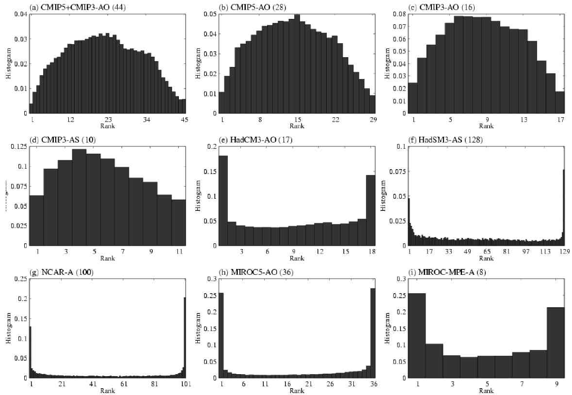
図 1 : マルチモデルアンサンブル (CMIP5+CMIP3-AO, CMIP3-AO, CMIP3-AS) および物理パラメータアンサンブル (HadCM3-AO, HadSM3-AS, NCAR-A, MIROC5-AO) マルチ物理スキームアンサンブル (MIROC-MPE-A) の順位頻度分布。気候場として、地表気温・降水量・海面気圧・大気上端における短波放射・長波放射の全天・晴天・雲放射強制力を利用した。横軸は順位で、最小値が 1 位、最大値がモデルアンサンブルメンバー数+1。縦軸は順位の頻度を表す。
