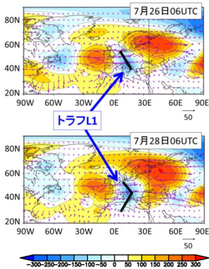
図 16 250hPa における高度場偏差の低周波変動成分(色塗り;単位は m)と波活動度フラックス(ベクトル;単位は m^2/s^2 )。JRA-25/JCDAS データの解析結果。波活動度フラックスは Takaya and Nakamura (2001) に基づく。
