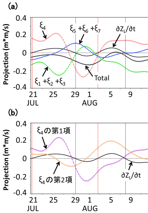
図 8 250hPa におけるロシア域 (32.5°E~62.5°E, 50°N~70°N)での渦度収支バランス。(a) 高度場変化傾向 \partial Z_L / \partial t , 全収支項 \sum_{i=1}^7 \xi_i , 移流項 \sum_{i=1}^3 \xi_i , 発散項 \xi_4 , 非線形項 \sum_{i=5}^7 \xi_i の時間変動。(b) 高度場変化傾向 \partial Z_L / \partial t , 発散項 \xi_4 の第 1 項, 第 2 項の時間変動。ただし, 各項は式(7)により, ロシア域の平均高度場偏差(図 7a)に射影した値を示す。
