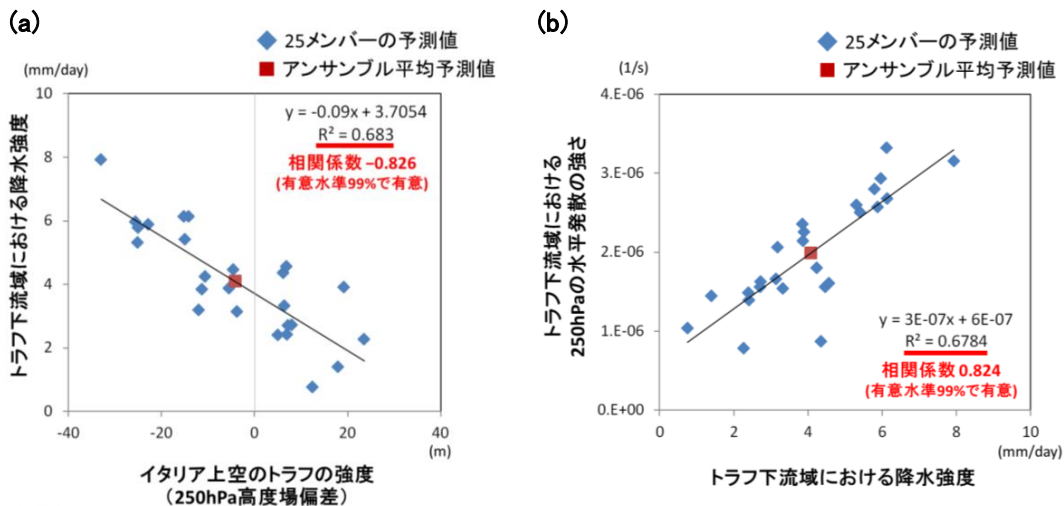
図13 (a) 2010年7月24日におけるイタリア上空( 10^{\circ}\text{E} \sim 25^{\circ}\text{E} , 35^{\circ}\text{N} \sim 50^{\circ}\text{N} )のトラフ強度の予測値とその下流域( 20^{\circ}\text{E} \sim 30^{\circ}\text{E} , 40^{\circ}\text{N} \sim 50^{\circ}\text{N} )における平均降水量の予測値との相関。ただし、2010年7月21日12UTCを予報初期時刻とする気象庁現業1か月アンサンブル予報データ(メンバー数25)を用いて解析した。トラフ強度は領域平均した250hPa高度場偏差の低周波変動成分(日平均値)、平均降水量は24時間積算降水量の領域平均値で定義した。(b) 同時刻におけるトラフ下流域( 20^{\circ}\text{E} \sim 30^{\circ}\text{E} , 40^{\circ}\text{N} \sim 50^{\circ}\text{N} )の平均降水量と、同じ領域で平均した250hPaでの水平発散との相関。用いた予報結果と、平均降水量の定義は図13aに同じ。
