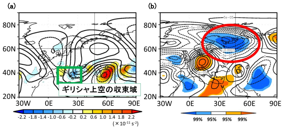
図 15 2010年8月5日 06UTCにおけるギリシャ域 C_G (10°E～35°E, 30°N～45°N) で平均した 250hPa 等圧面での渦度ソース S_{42} \equiv -\zeta_L \nabla \cdot \vec{V} の値と、同時刻における高度場変化傾向 \partial Z_L / \partial t との回帰分析。2010年7月28日 12UTC を予報初期時刻とする気象庁現業 1 か月アンサンブル予報データ (メンバー数 25) を用いた。(a) 250hPa における渦度ソース S_{42} (色塗り) と高度場偏差 Z_L (等値線; 等値線間隔は 50m) のアンサンブル平均予測場。寒色 (暖色) は高気圧性 (低気圧性) 渦度生成を表す。(b) \partial Z_L / \partial t の回帰場 (等値線; 等値線間隔は 2.5 \times 10^{-5} m/s)。Student-t テストにより求めた相関係数の統計的有意性が 95% 以上の領域に色塗りをした。寒色 (暖色) は負 (正) の相関を示す。
