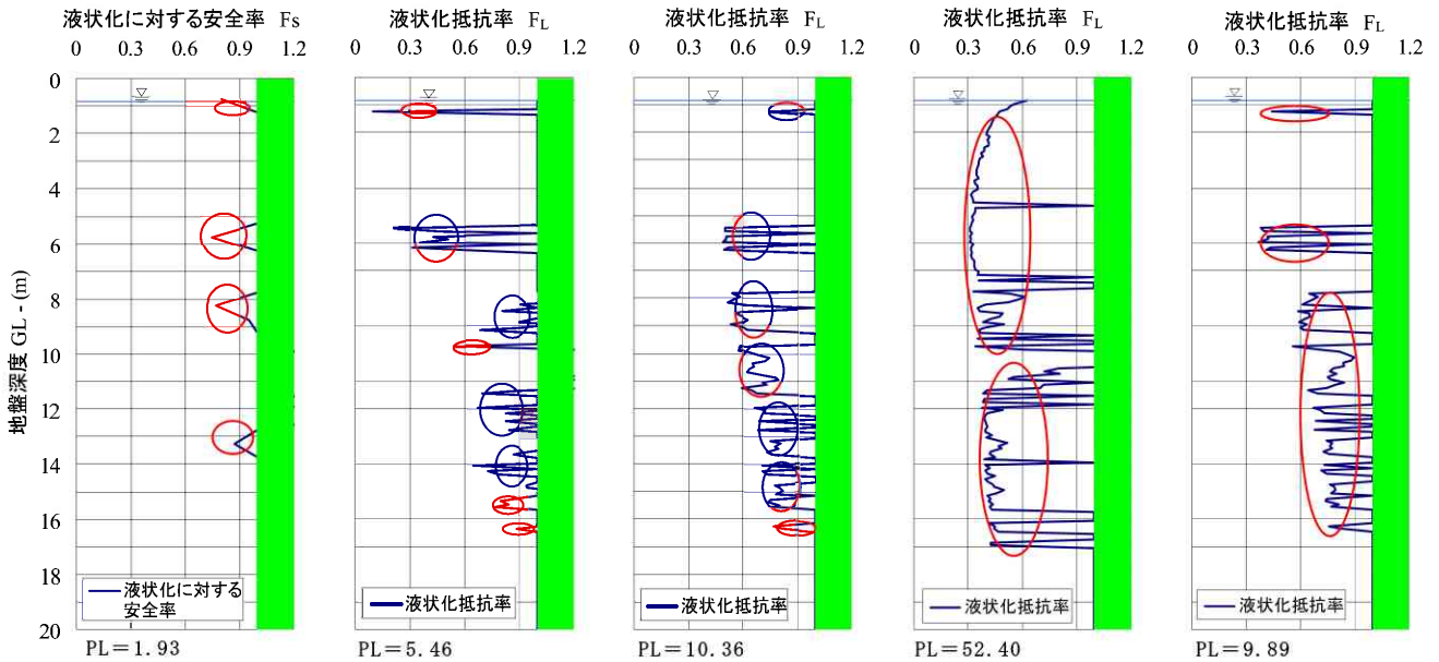
図-5(b) RI コーン貫入試験結果に基づいて、5 種類の手法によって算定した液状化危険度評価結果
