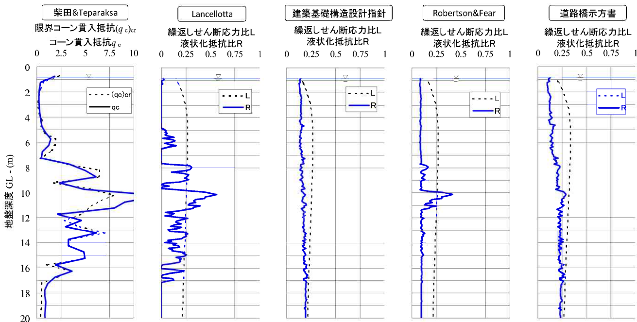
図-5(a) RI コーン貫入試験結果に基づいて算定した、5種類の手法による液化化抵抗値 R と地震によって動員される繰り返しせん断応力比 L の深度方向分布
