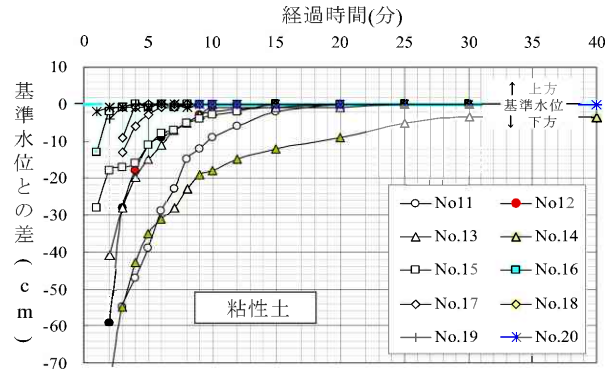
図-3 (b) 測定水位と経過時間(粘性土の結果)
