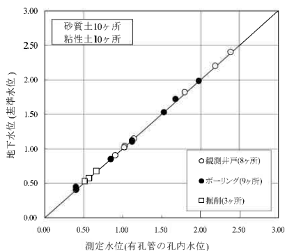
図-2 地下水位（基準水位）と有孔管の孔内水位との関係
