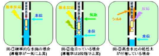
図-1 交流式比抵抗水位計による測定
