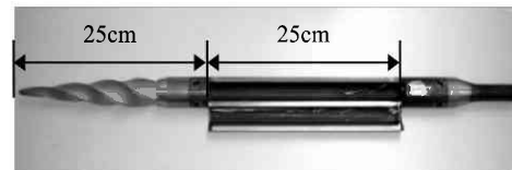
写真-4 土質試料採取器
